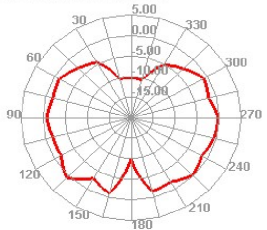
2500.000MHz E2
