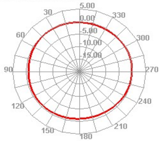
2500.000MHz H
