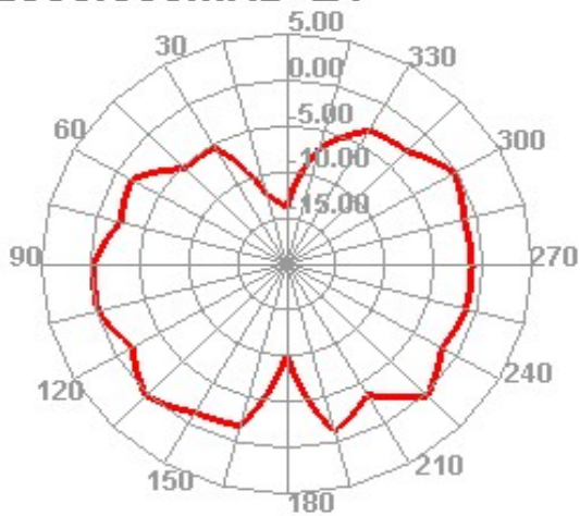
2500.000MHz E1
