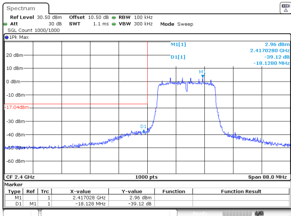
802.11n20_2412MHz
