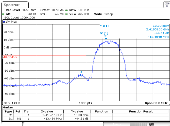
802.11b_2412MHz
