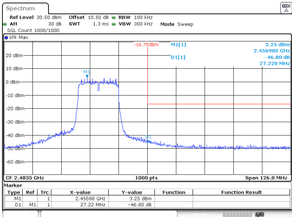
802.11n20_2462MHz
