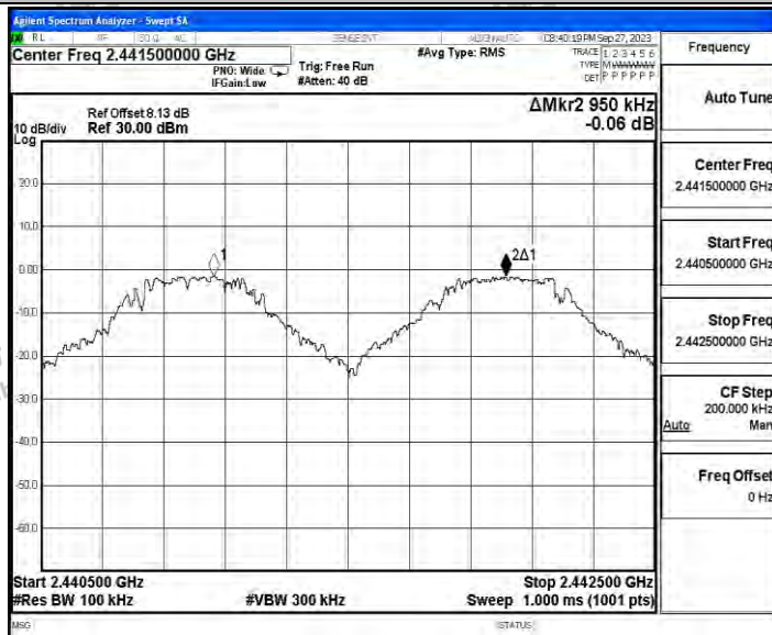
2DH5_Ant_Hop
