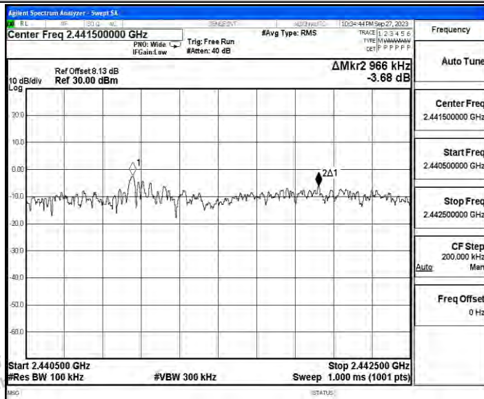
3DH5_Ant_Hop
