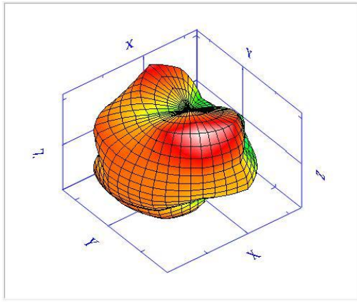
2440MHz
