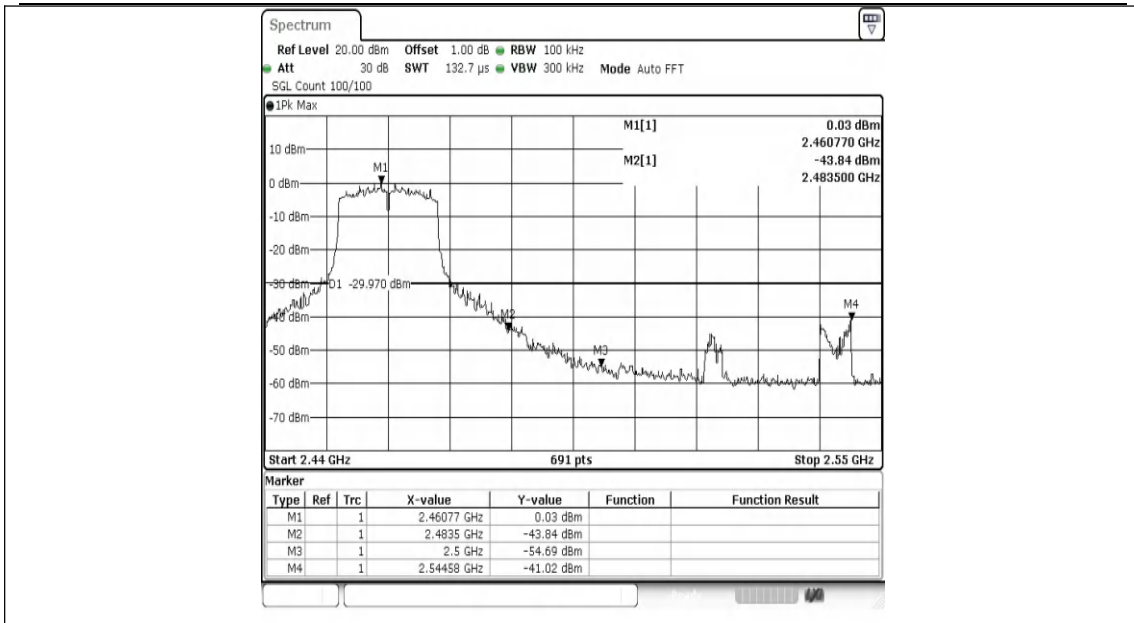
11N20MIMO-Ant0-2462-PASS
