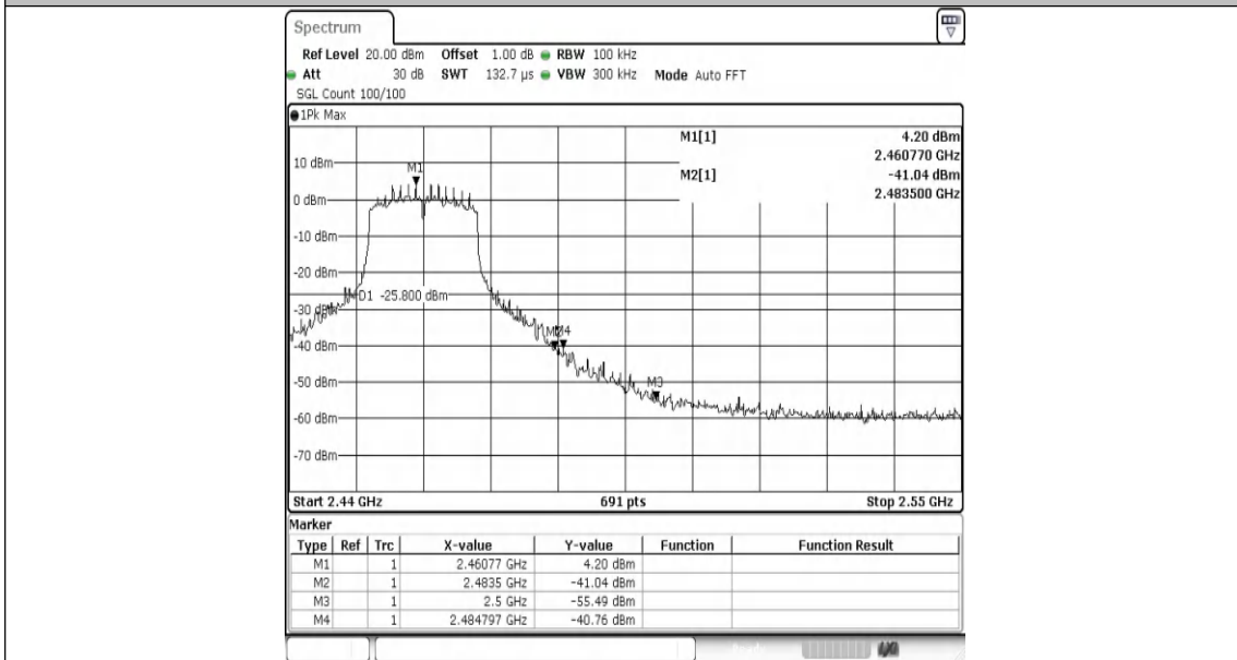
11N20MIMO-Ant0-2462-PASS
