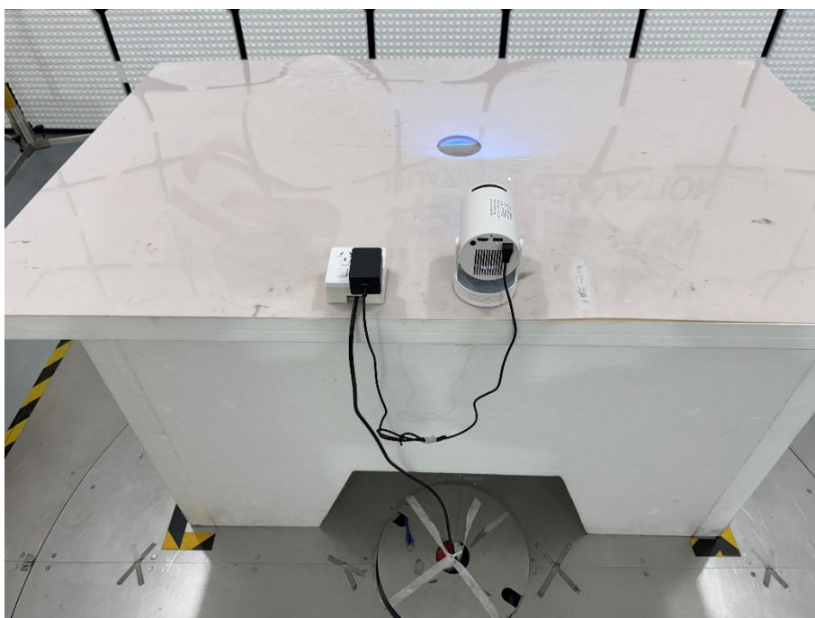
30MHz - 1GHz - 2
