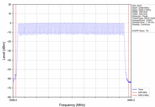
Pi/4DQPSK_2DH5_HOPP_Ant1_NTNV
