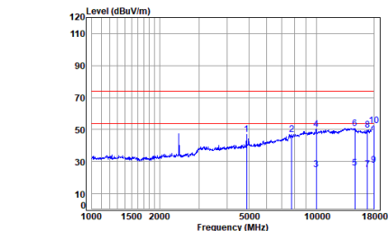
BT_DH5_TX_CH_39_Horizontal
