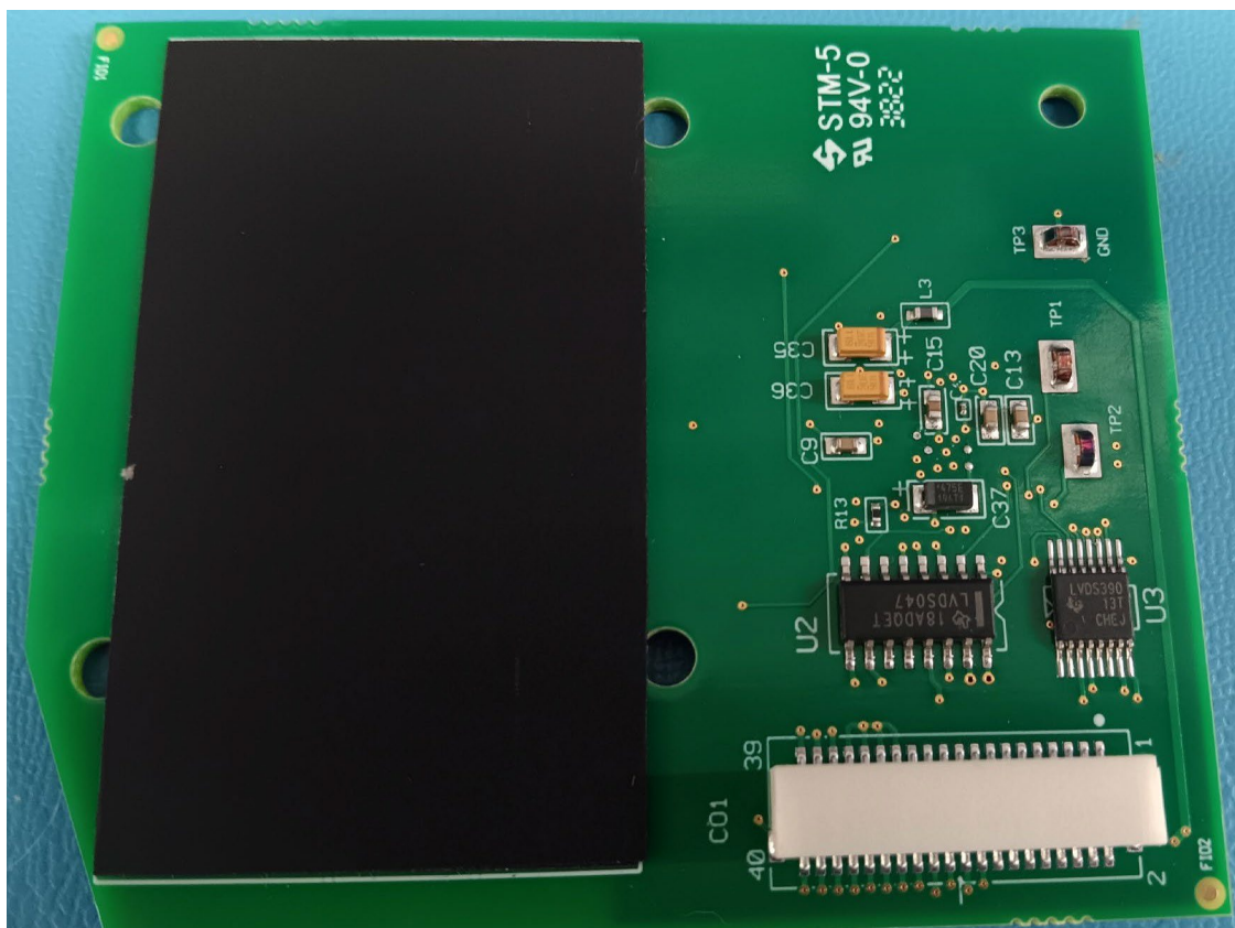
NFC Side 2
