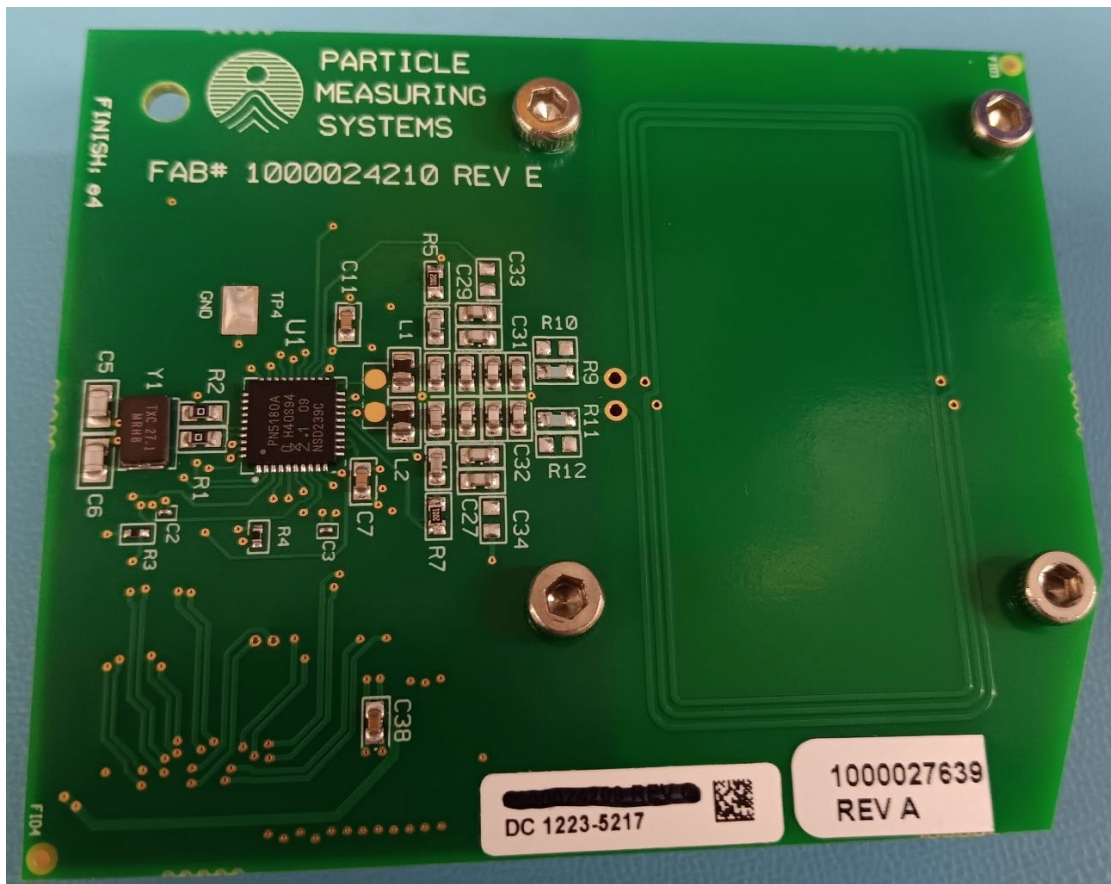
NFC Side 1
