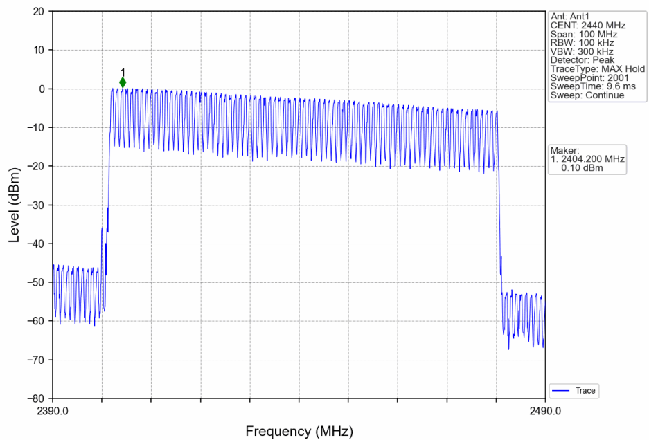
GFSK_DH5_HOPP_2404MHz_Ant1_NTNV
