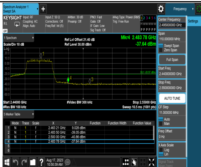
11AX20MIMO_Ant2_High_2462
