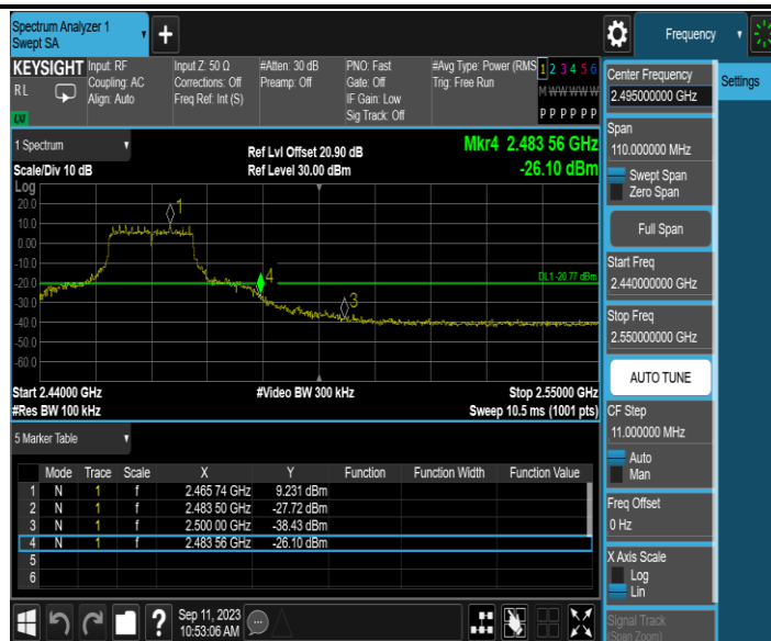
11N20MIMO_Ant2_High_2462
