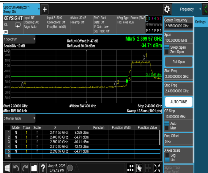
11N20MIMO_Ant2_Low_2412
