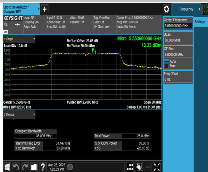
11AC40MIMO_Ant2_5550
