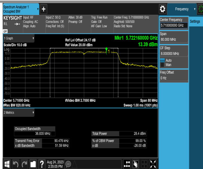
11AC40MIMO_Ant2_5710
