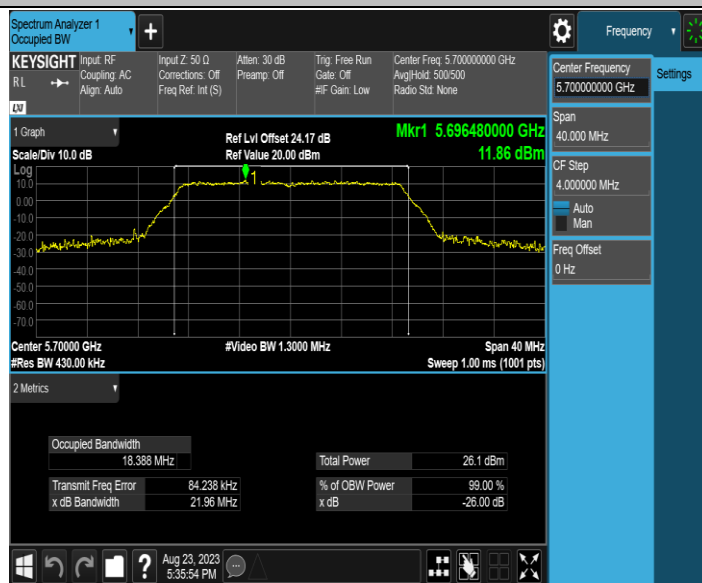
11AC20MIMO_Ant2_5700
