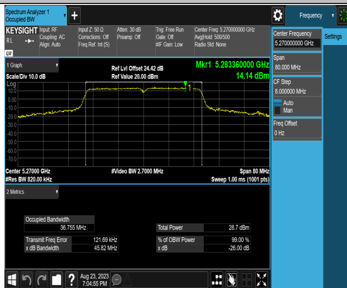
11AC40MIMO_Ant2_5270
