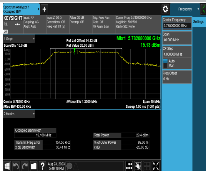
11AC20MIMO_Ant2_5785
