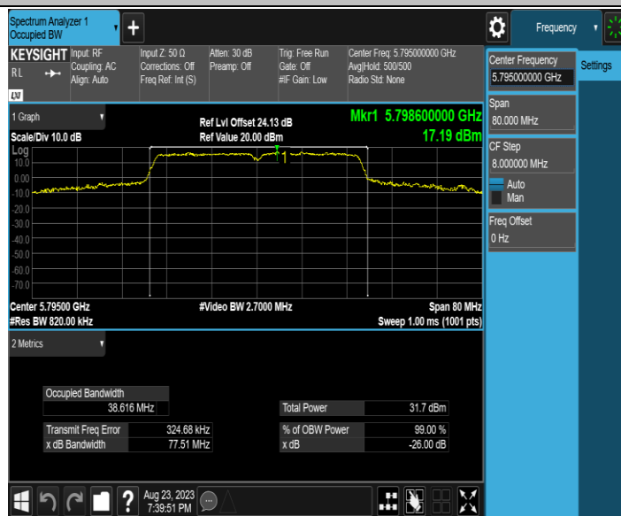
11AC40MIMO_Ant2_5795
