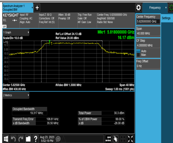
11AC20MIMO_Ant2_5825
