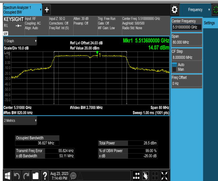
11AC40MIMO_Ant2_5510
