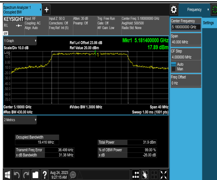
11AX20MIMO_Ant2_5180
