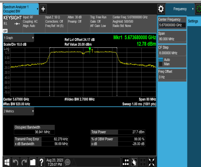
11AC40MIMO_Ant2_5670
