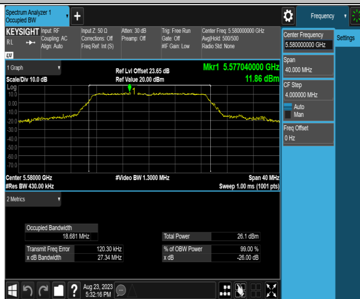
11AC20MIMO_Ant2_5580
