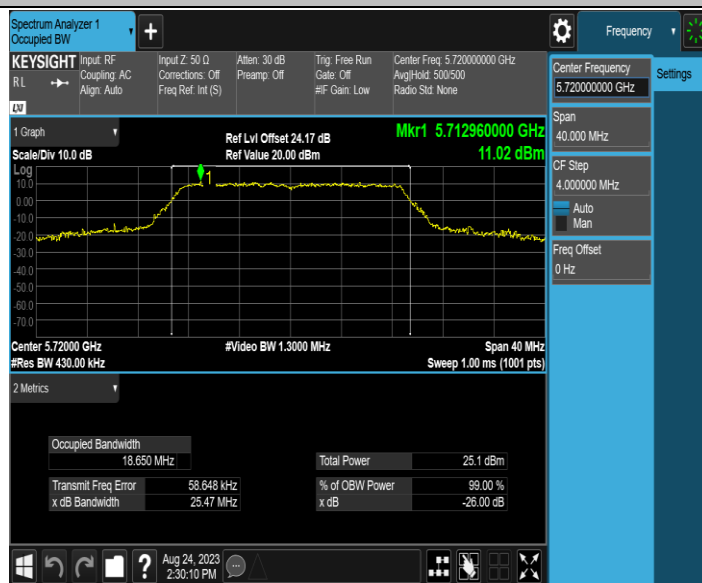
11AC20MIMO_Ant2_5720
