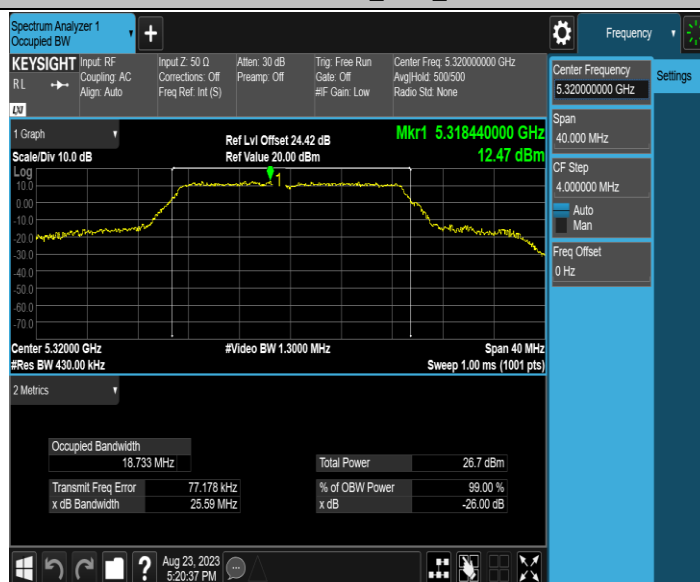
11AC20MIMO_Ant2_5320
