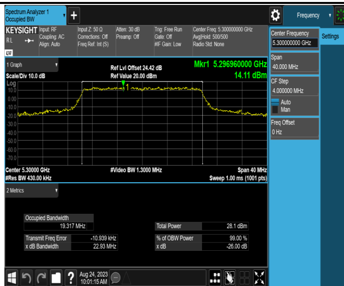
11AX20MIMO_Ant2_5300
