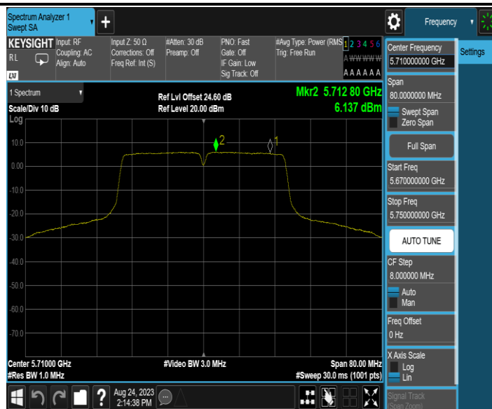
11N40MIMO_Ant2_5710_UNII-2C
