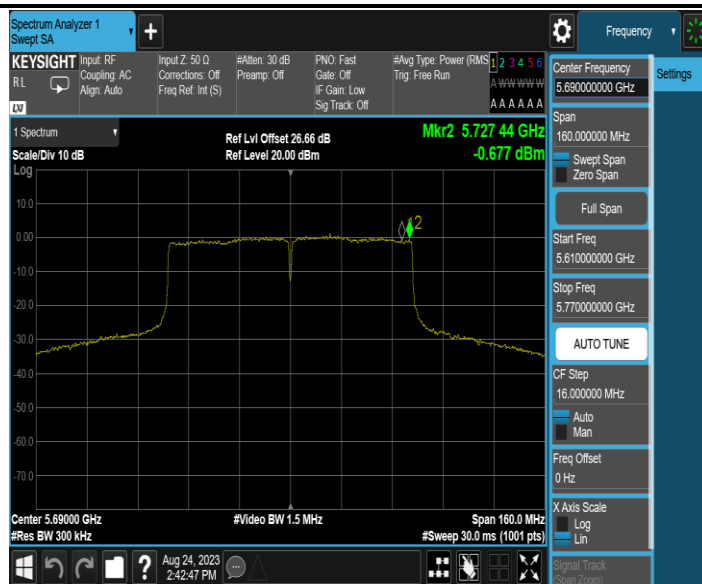
11AC80MIMO_Ant2_5690_UNII-3
