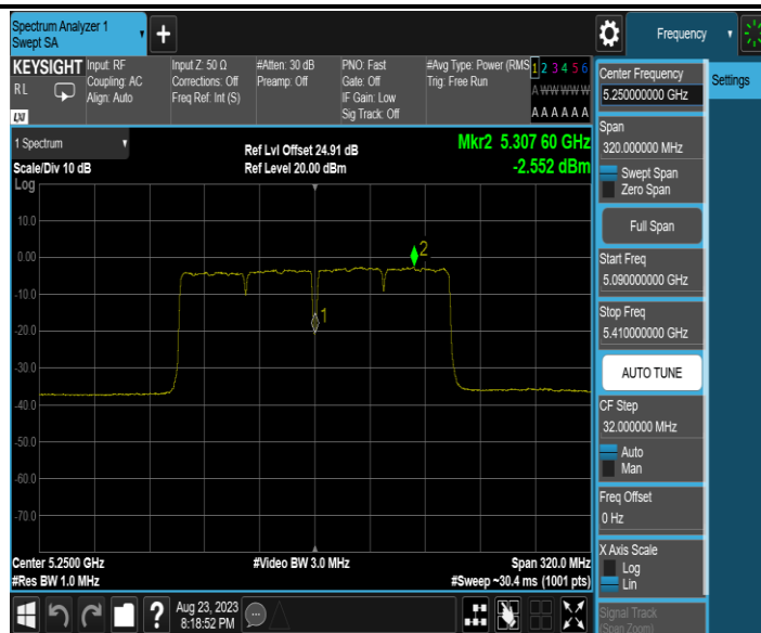
11AC160MIMO_Ant2_5250_UNII-2A
