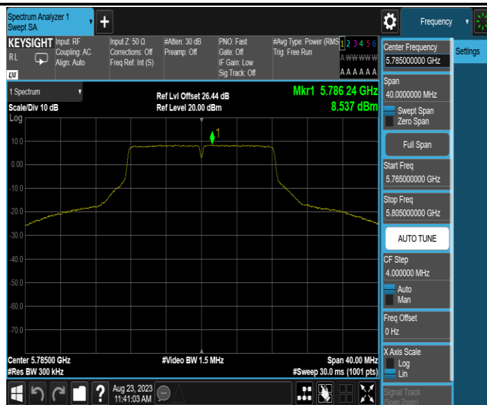
11A_Ant2_5785
