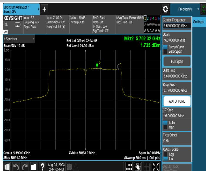
11AC80MIMO_Ant1_5690_UNII-3
