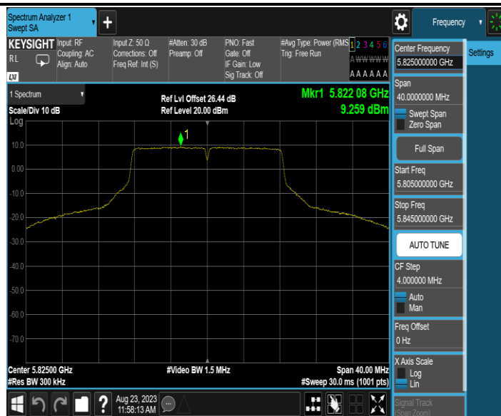
11A_Ant2_5825
