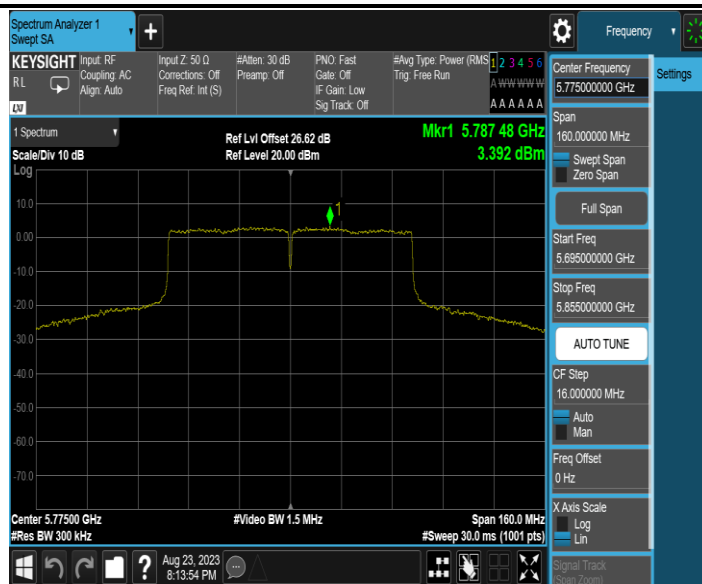
11AC80MIMO_Ant2_5775
