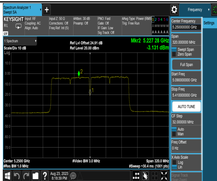
11AC160MIMO_Ant2_5250_UNII-1
