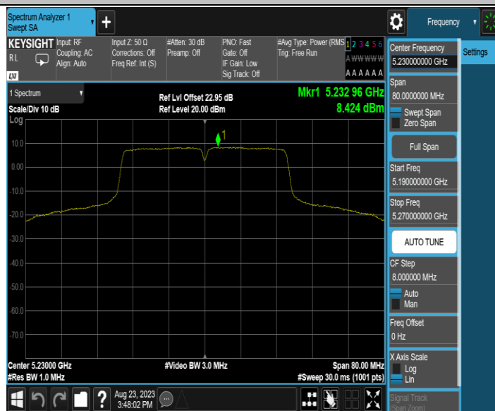
11N40MIMO_Ant1_5270
