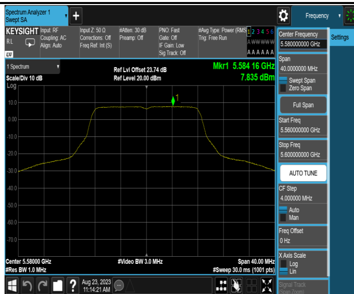
11A_Ant2_5580
