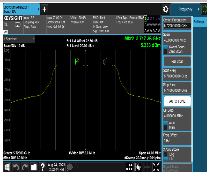
11A_Ant1_5720_UNII-3
