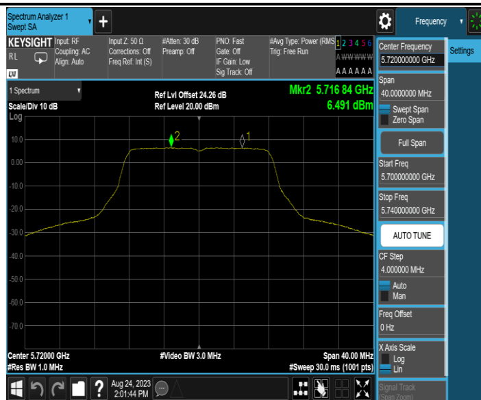
11A_Ant2_5720_UNII-2C
