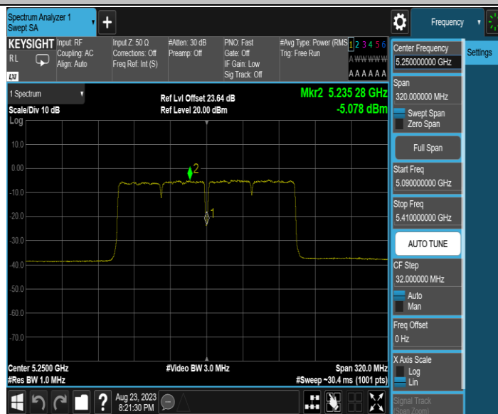
11AC160MIMO_Ant1_5250_UNII-2A
