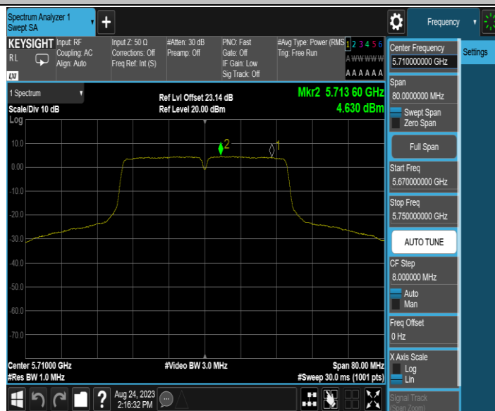
11N40MIMO_Ant1_5710_UNII-3
