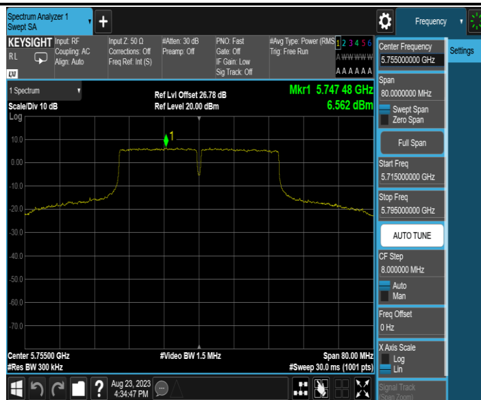
11N40MIMO_Ant2_5755
