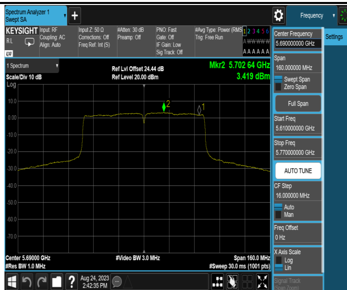
11AC80MIMO_Ant2_5690_UNII-2C
