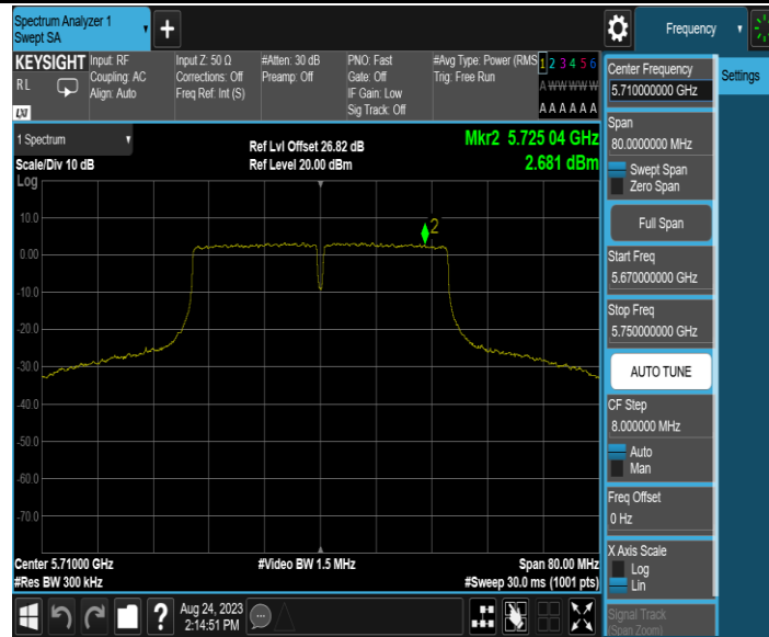
11N40MIMO_Ant2_5710_UNII-3
