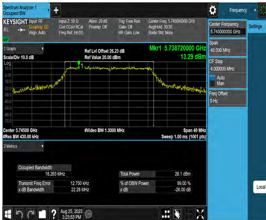
11N20MIMO_Ant4_5745
