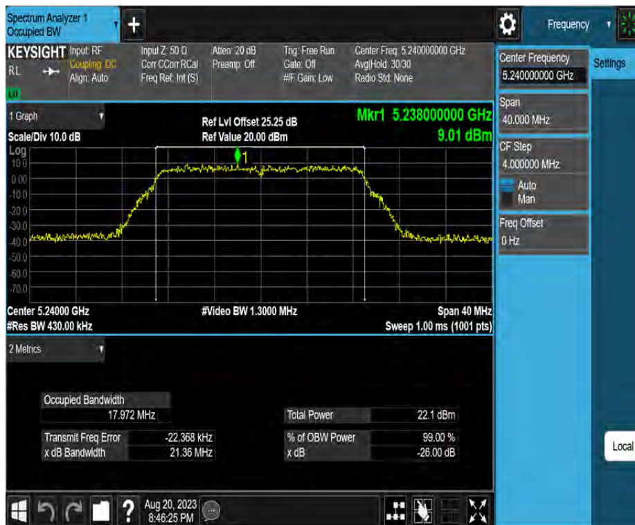
11N20MIMO_Ant4_5240
