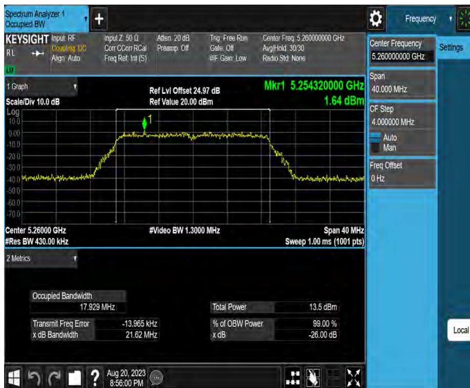
11N20MIMO_Ant2_5260
