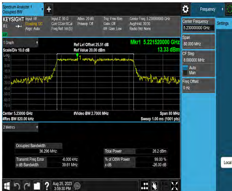
11N40MIMO_Ant2_5230
