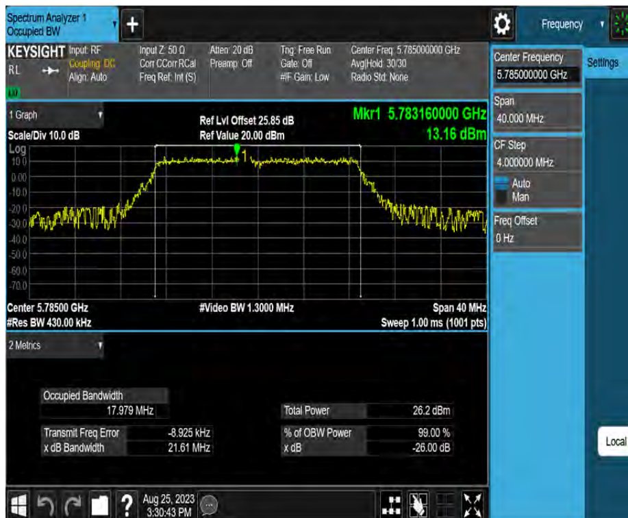
11N20MIMO_Ant4_5785
