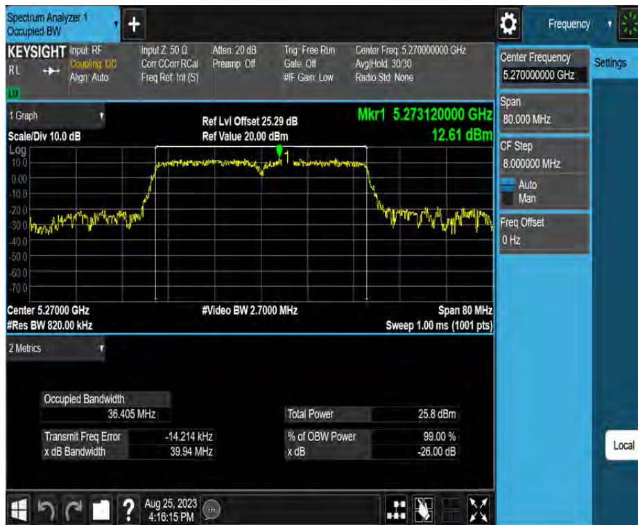
11N40MIMO_Ant4_5270
