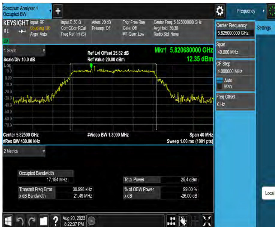
11A_Ant2_5825
