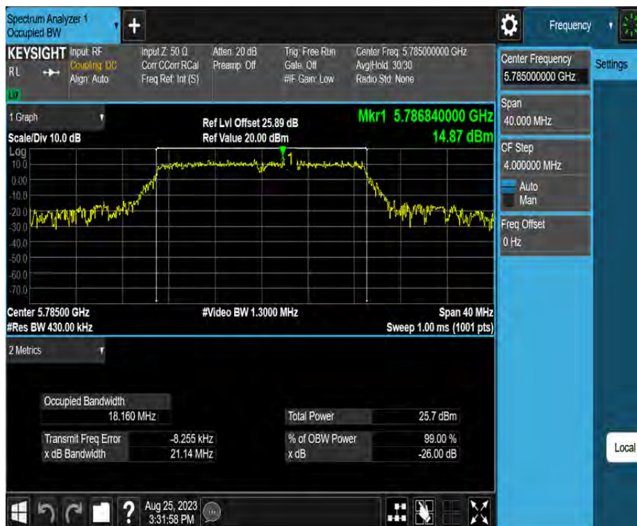
11N20MIMO_Ant4_5785
