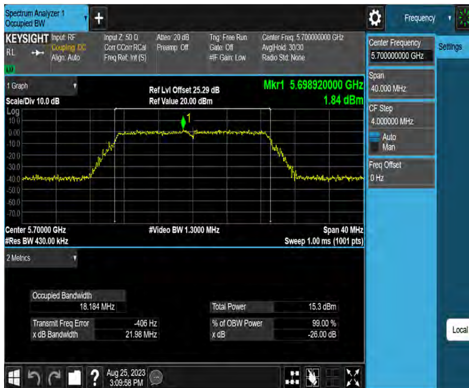
11N20MIMO_Ant2_5700
