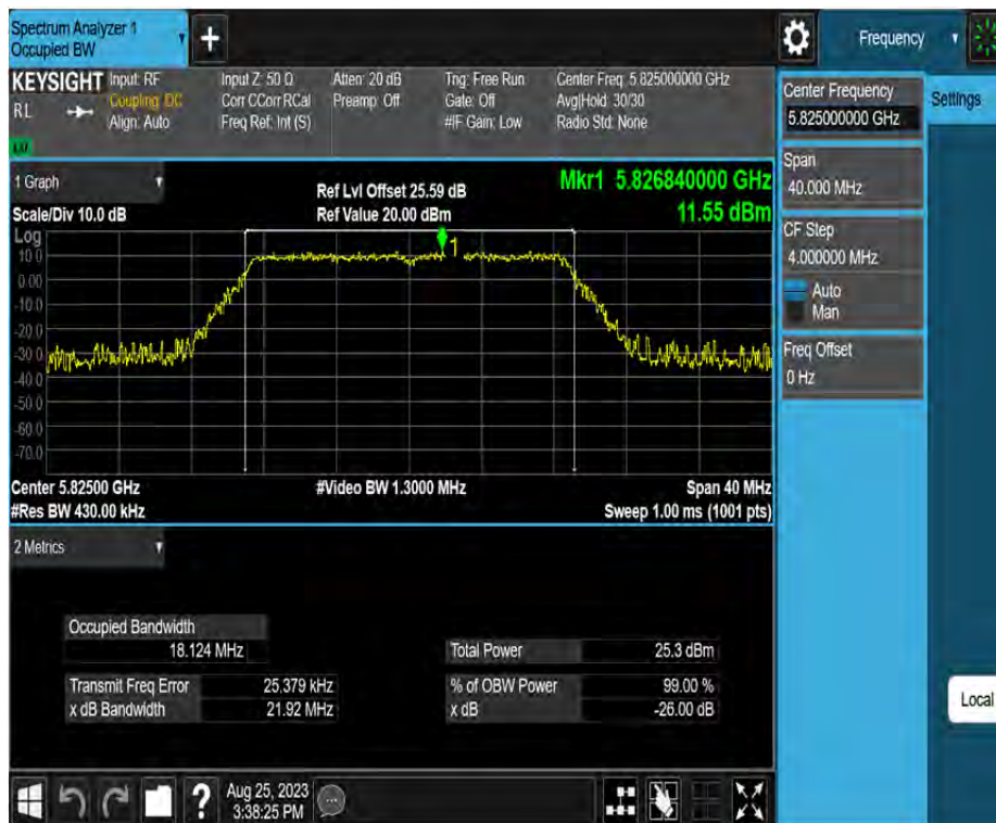
11N20MIMO_Ant2_5825
