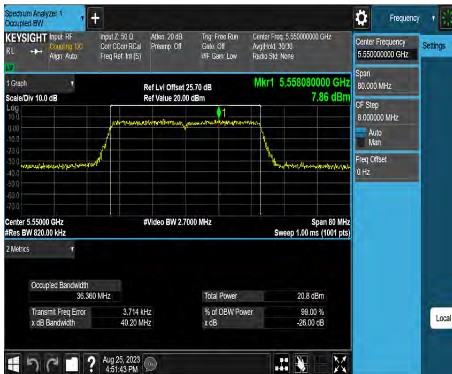
11N40MIMO_Ant4_5550
