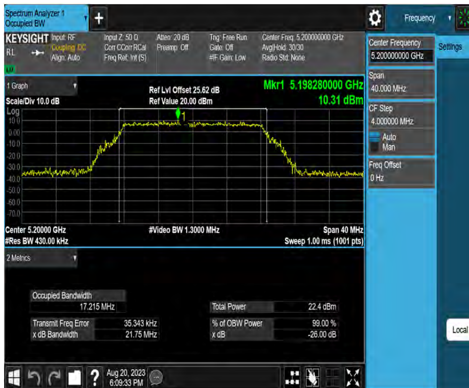
11A_Ant2_5200
