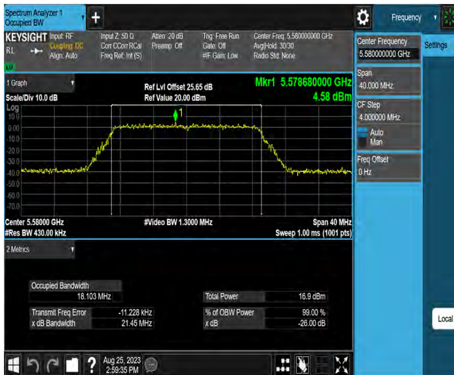
11N20MIMO_Ant4_5580
