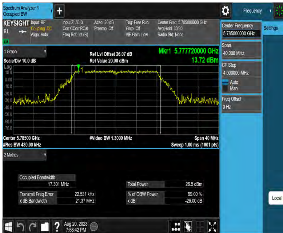
11A_Ant2_5785
