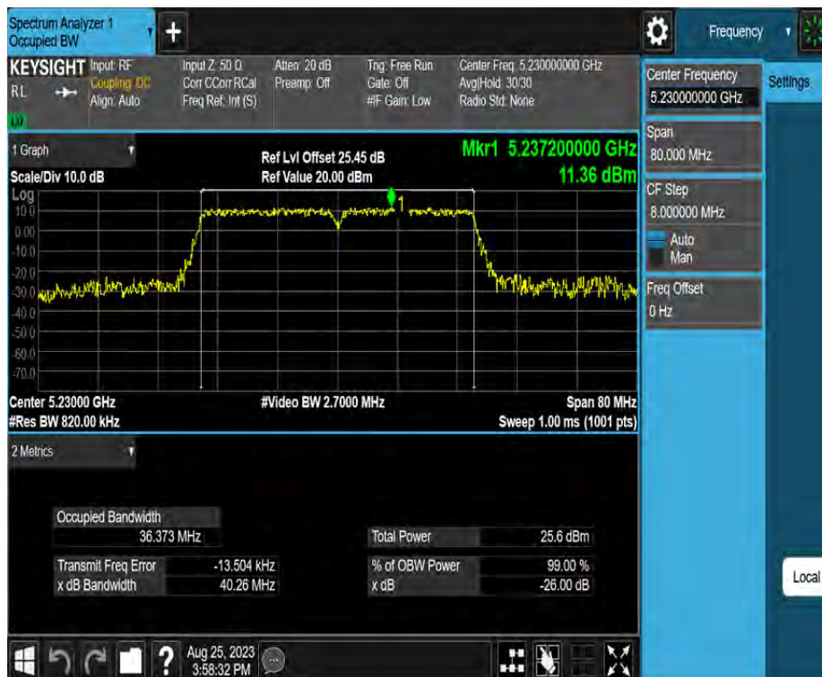
11N40MIMO_Ant2_5230
