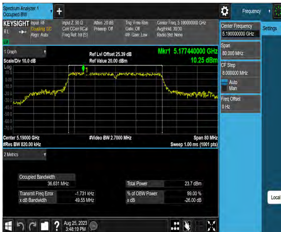
11N40MIMO_Ant4_5190
