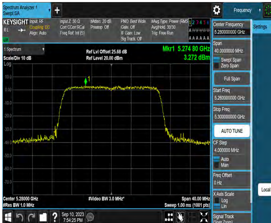
11AX20MIMO_Ant4_5280
