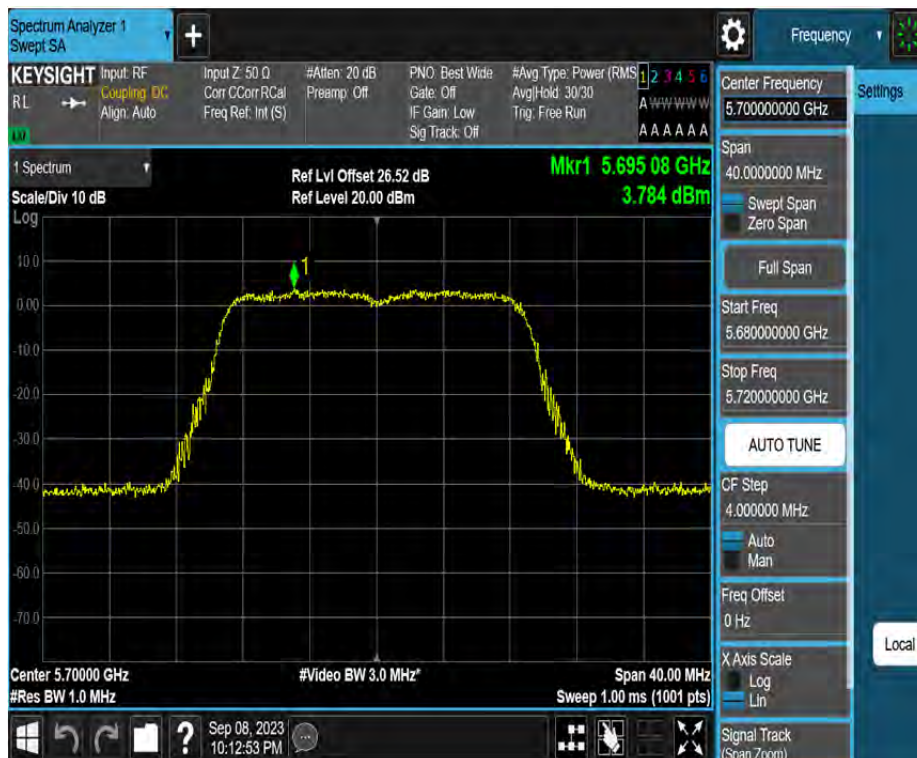
11AC20MIMO_Ant4_5700
