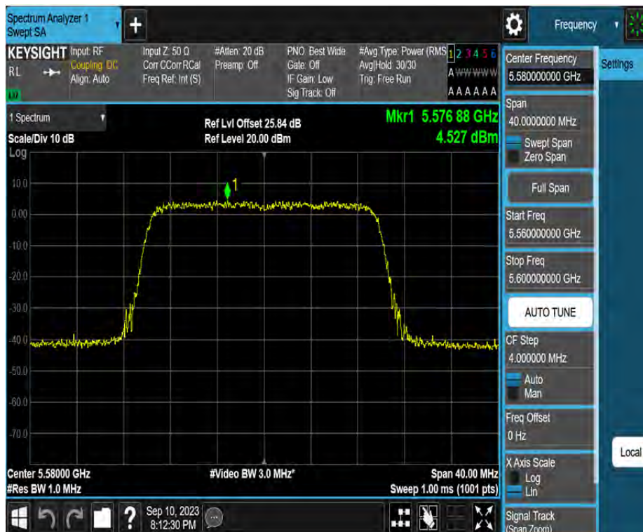
11AX20MIMO_Ant2_5580
