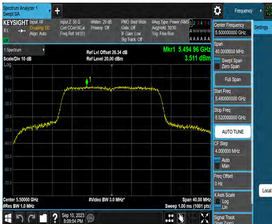
11AX20MIMO_Ant4_5500
