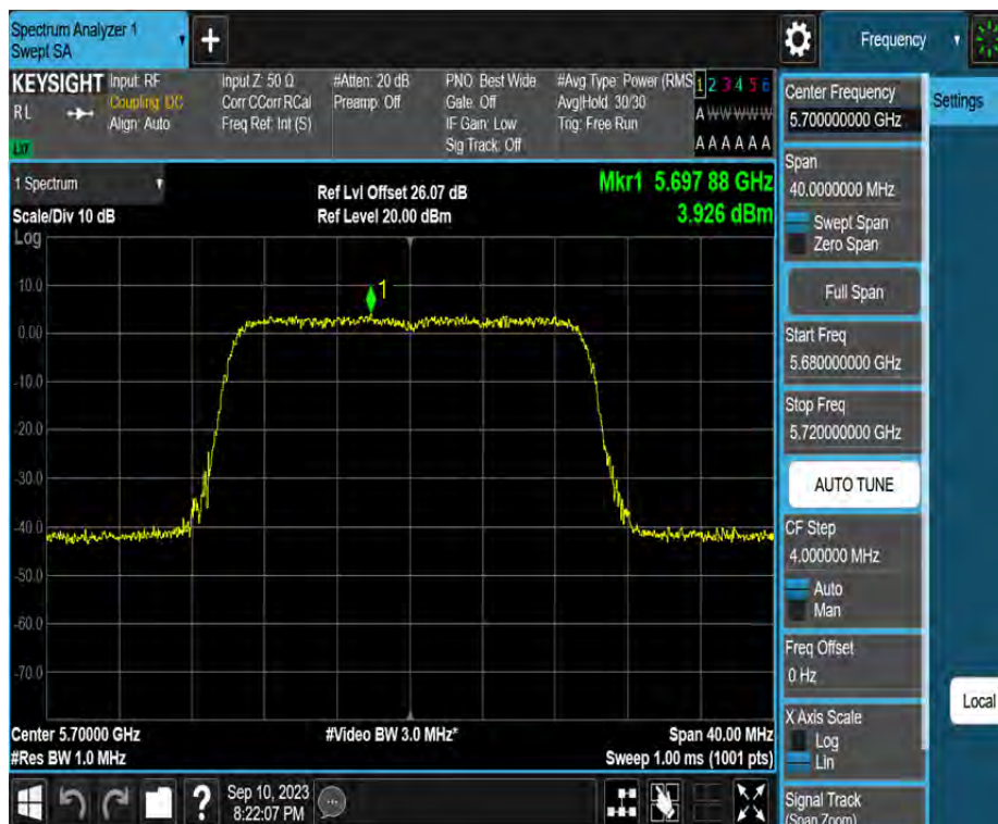
11AX20MIMO_Ant2_5700
