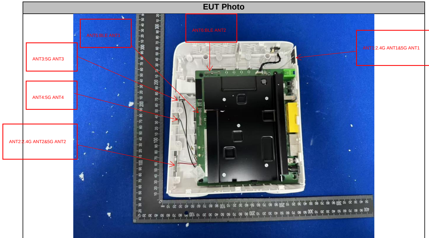
EUT Photo
