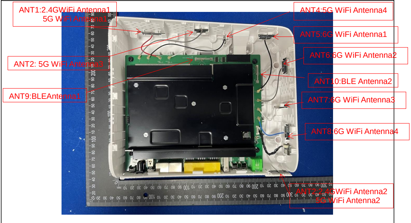
EUT Photo
