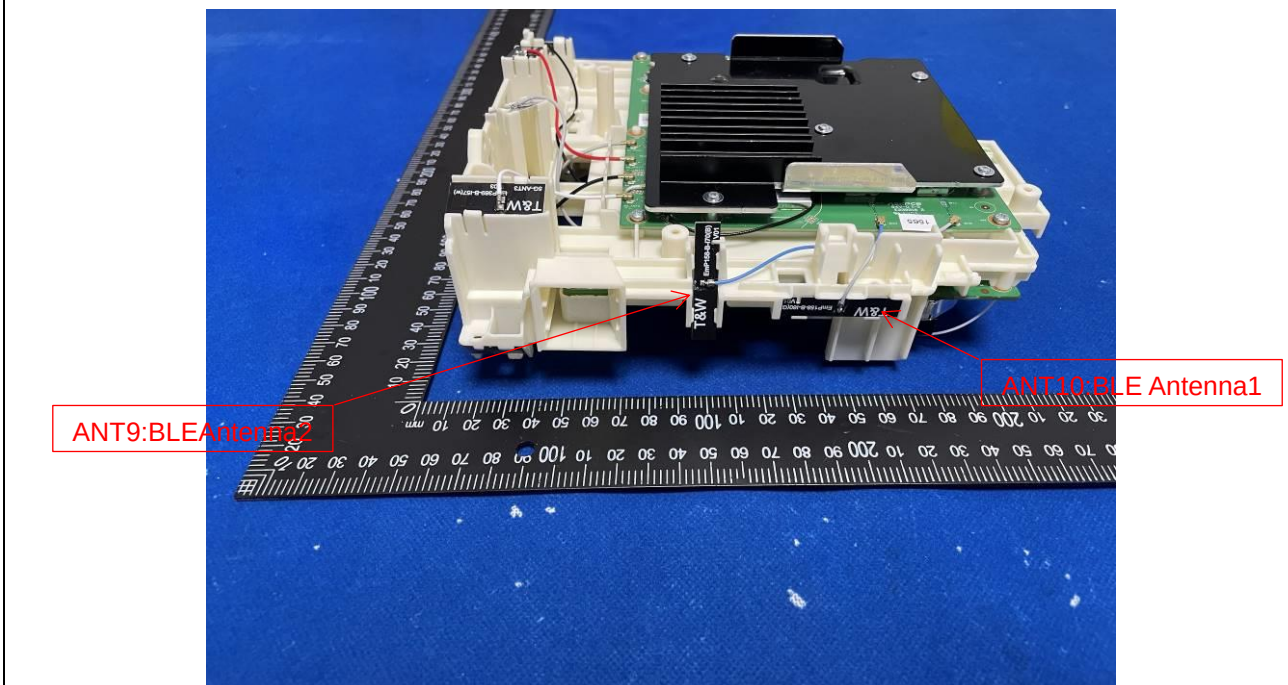
EUT Photo
