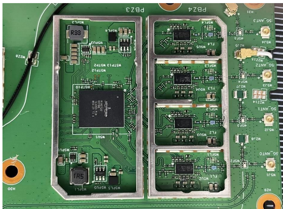
EUT Photo
