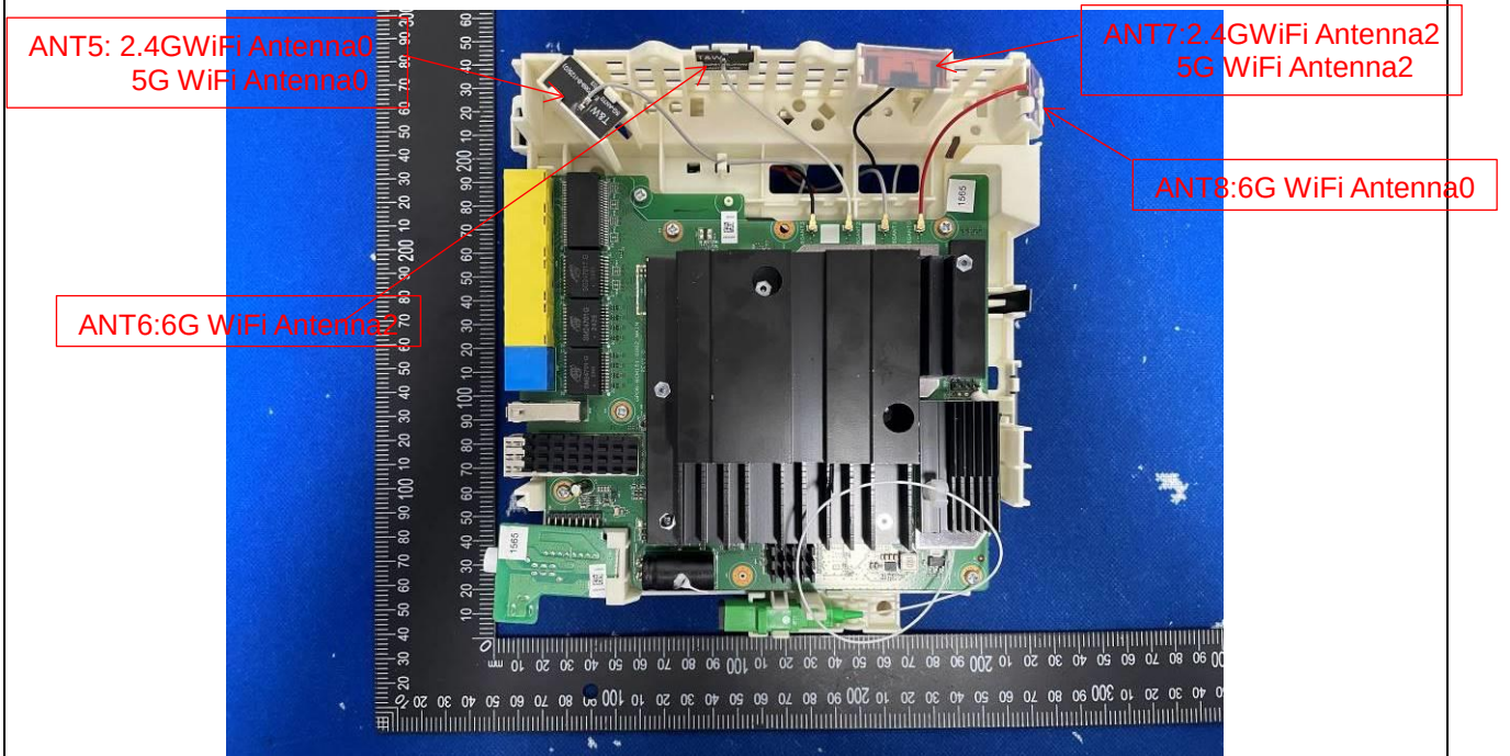
EUT Photo
