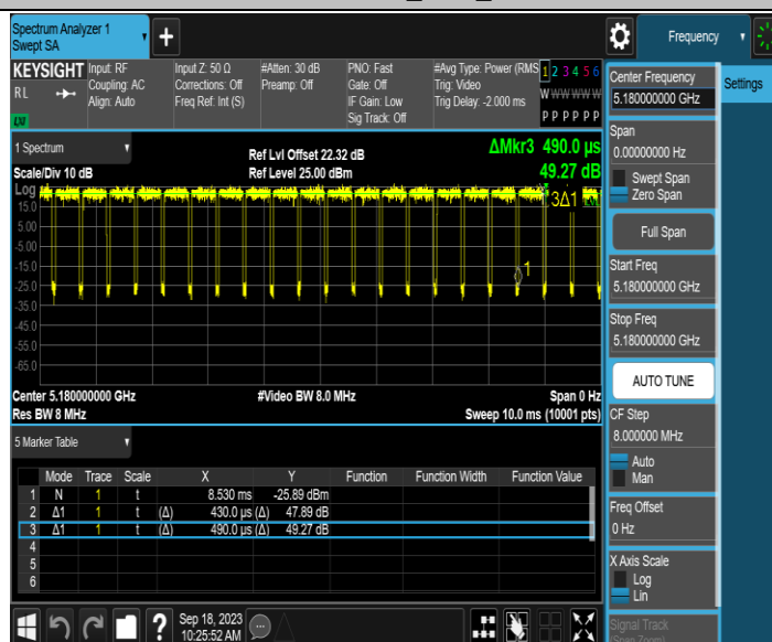
11AX40MIMO_Ant1_5190
