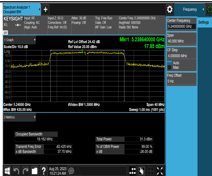
11AX20MIMO_Ant2_5240
