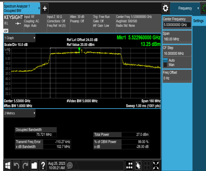
11AC80MIMO_Ant2_5530
