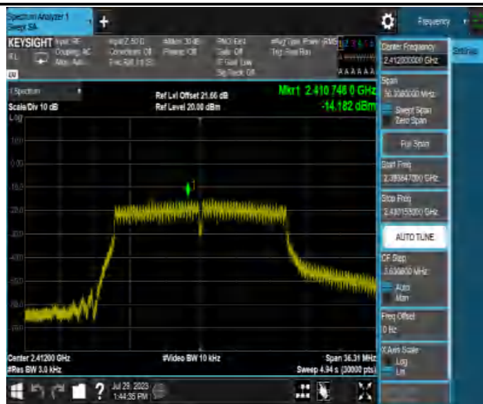
11N20MIMO_Ant2_2412
