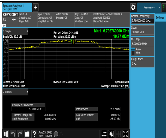
11AX40MIMO_Ant2_5795
