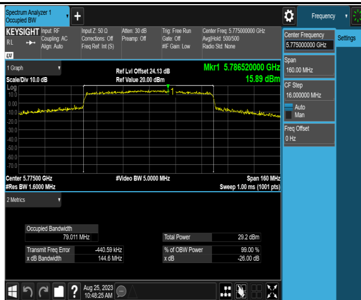
11AX80MIMO_Ant2_5775
