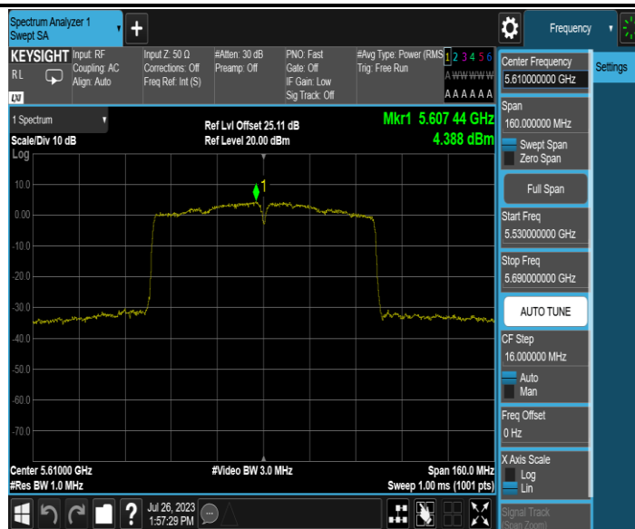
11AC80MIMO_Ant2_5610
