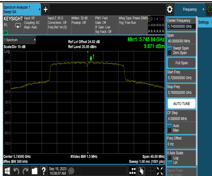
11AX20MIMO_Ant2_5745
