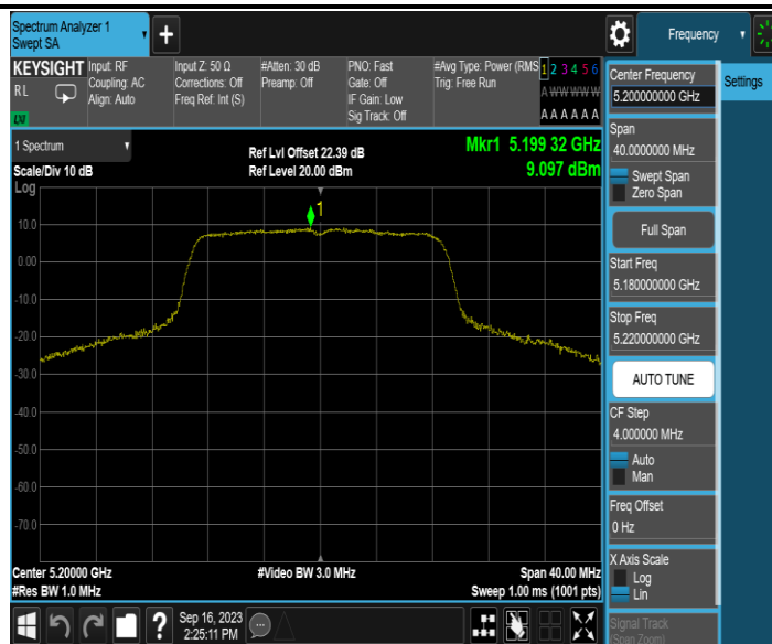
11AX20MIMO_Ant2_5200
