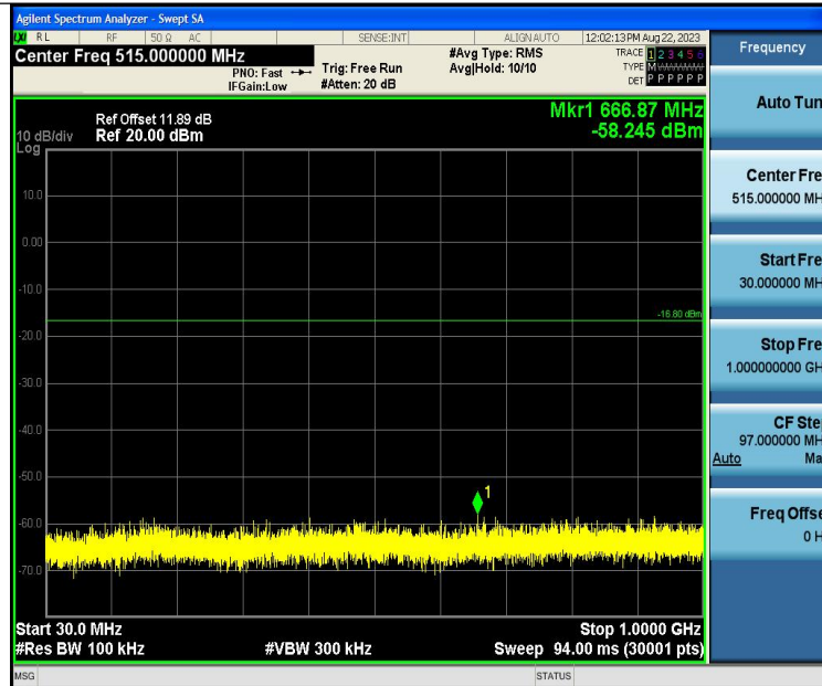
BLE_2M-Ant1-2402-30~1000-PASS
