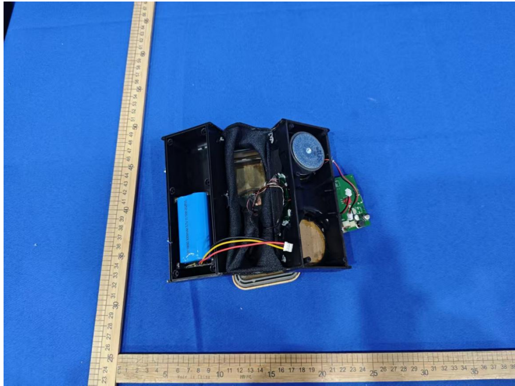
BT ANT
