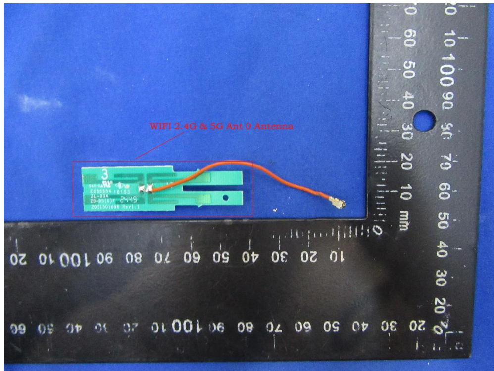
(10) EUT Photo (QPF4259)
