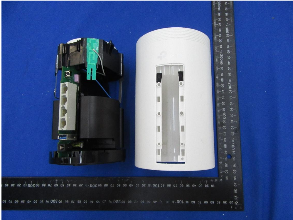
(4) EUT Photo (QPF4259)
