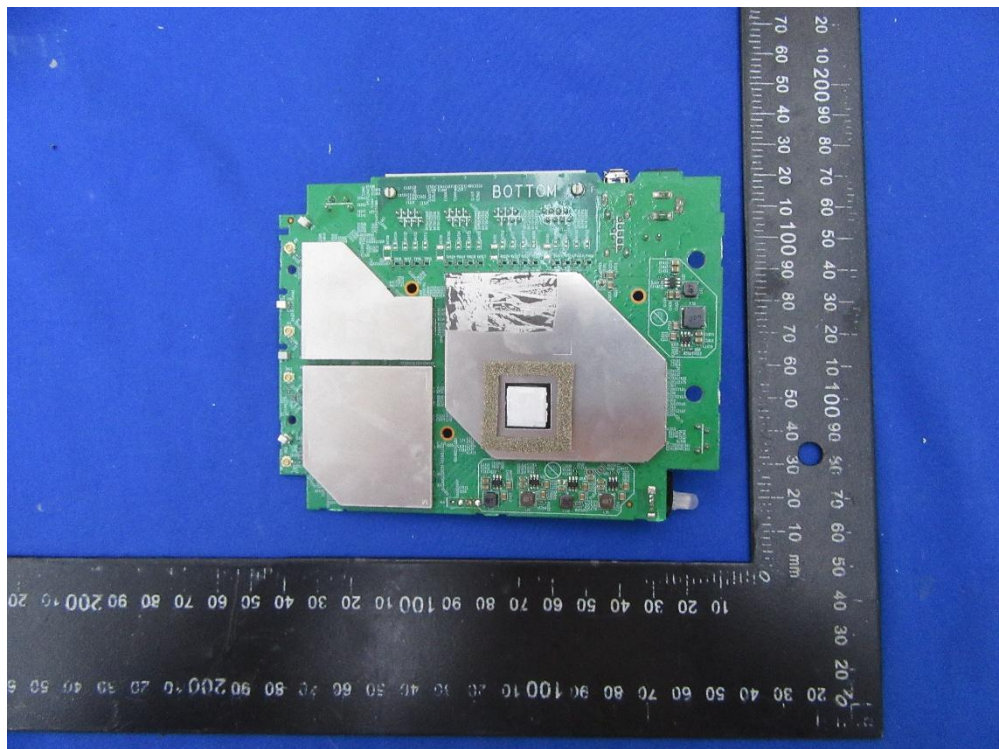
(14) EUT Photo (QPF4259)
