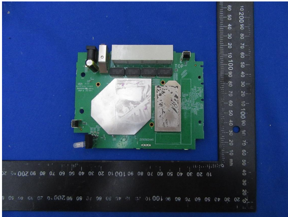
(16) EUT Photo (QPF4259)
