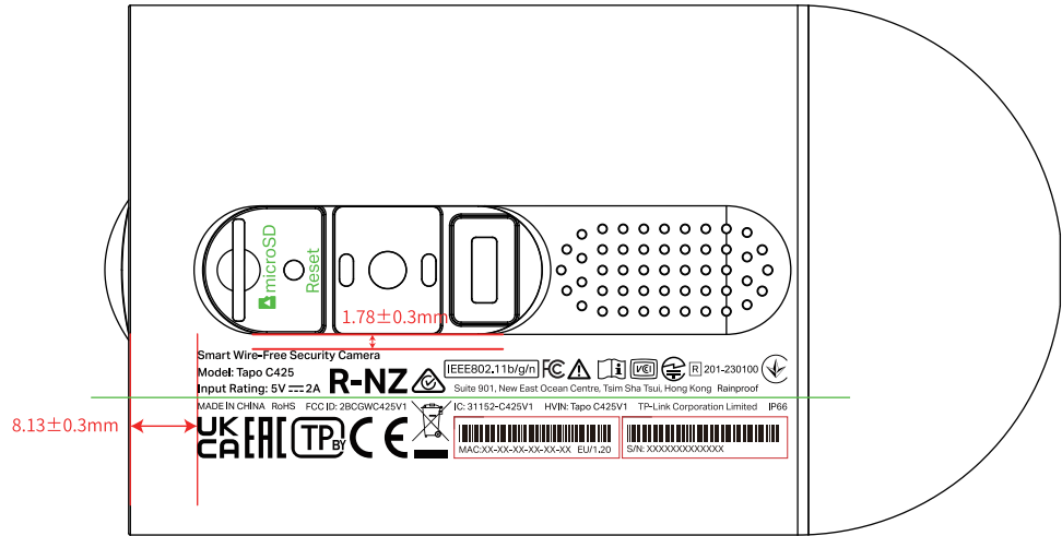
尺寸图
