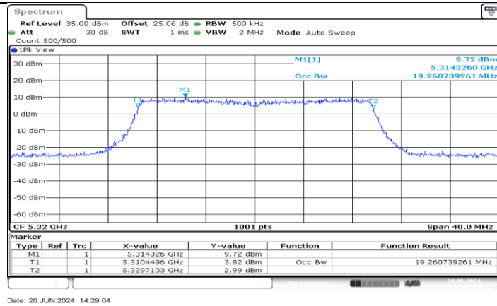
11AX20MIMO_Ant4_5320
