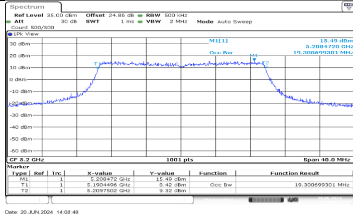
11AX20MIMO_Ant3_5200
