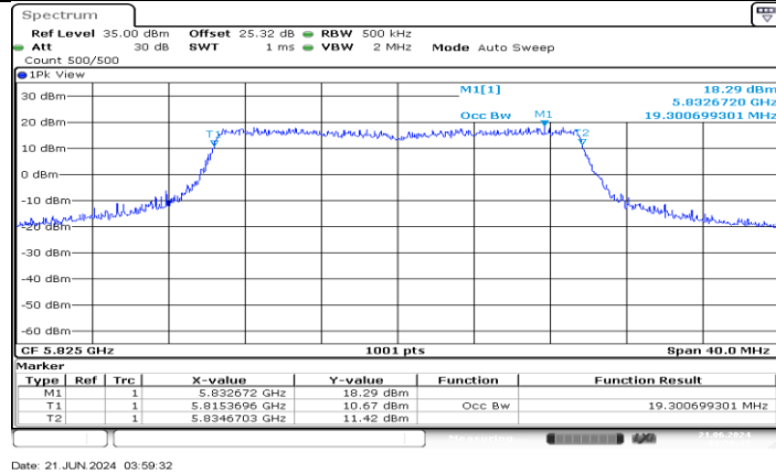
11AX20MIMO_Ant3_5825
