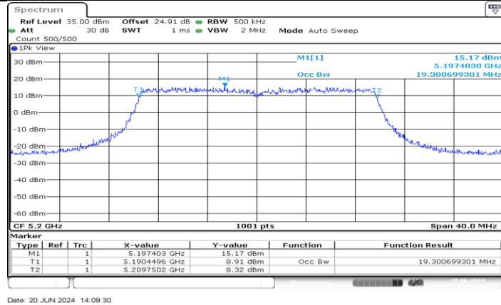
11AX20MIMO_Ant4_5200
