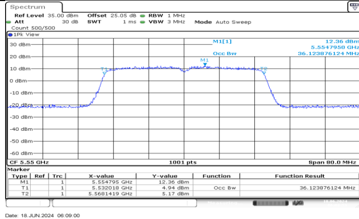
11AC40MIMO_Ant4_5550
