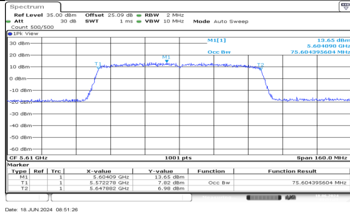
11AC80MIMO_Ant3_5610
