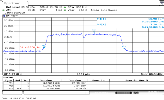
11AC40MIMO_Ant4_5270
