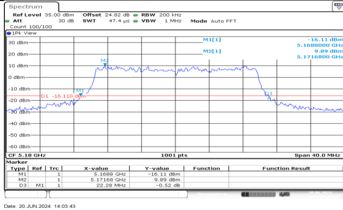
11AX20MIMO_Ant3_5180
