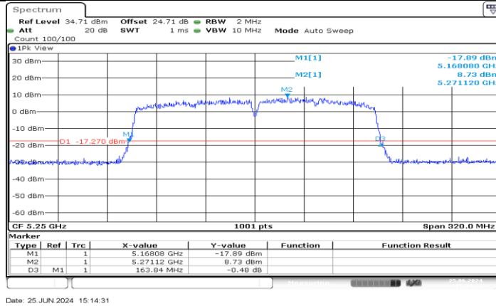
11AC160MIMO_Ant3_5250
