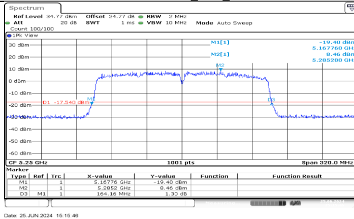
11AC160MIMO_Ant4_5250
