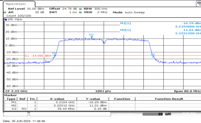
11AC40MIMO_Ant2_5230
