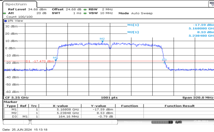
11AC160MIMO_Ant2_5250
