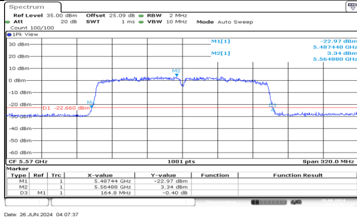
11AC160MIMO_Ant3_5570
