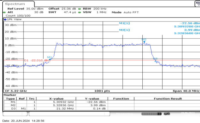
11AX20MIMO_Ant4_5320
