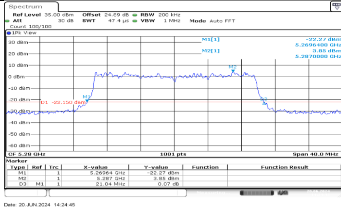
11AX20MIMO_Ant4_5280
