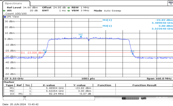
11AC80MIMO_Ant4_5530
