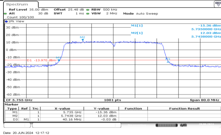
11AC40MIMO_Ant2_5755
