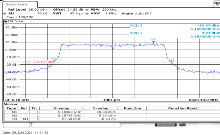
11AX20MIMO_Ant4_5180
