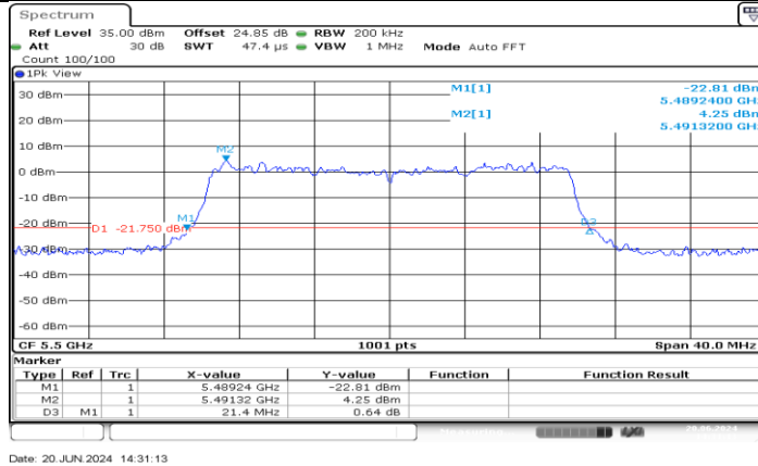
11AX20MIMO_Ant2_5500
