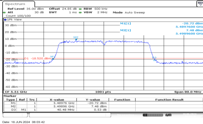
11AC40MIMO_Ant2_5510
