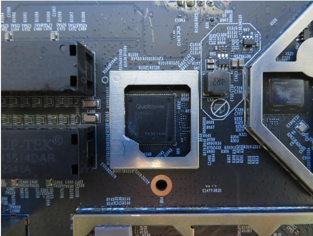
(17) EUT Phot 0
