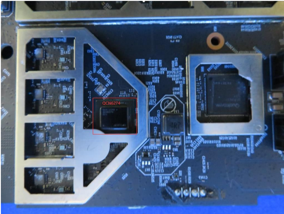
(18) EUT Phot 0
