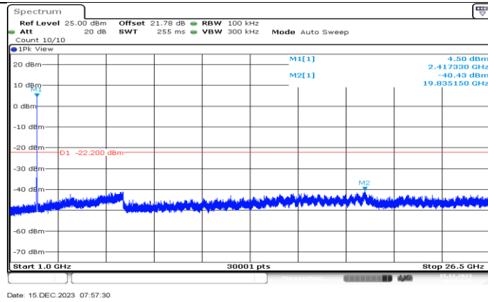
11G-CDD_Ant1_2417_1000~26500
