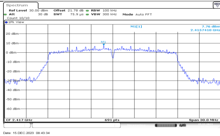
11N20MIMO_Ant1_2417_0~Reference
