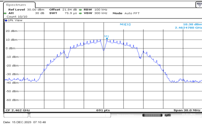
11B-CDD Ant1 2462 0~Reference
