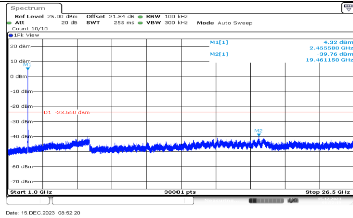
11N20MIMO_Ant1_2457_1000~26500
