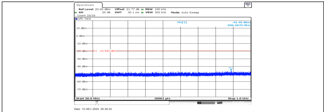
11B-CDD Ant2 2417 30~1000
