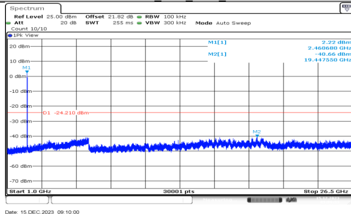
11N20MIMO_Ant2_2462_1000~26500
