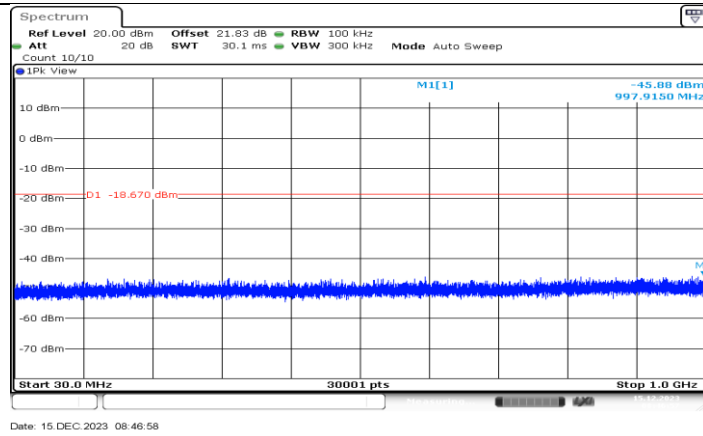
11N20MIMO Ant1 2437 30~1000
