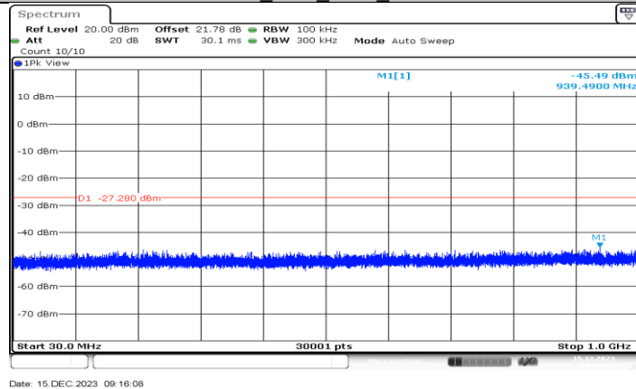
11N40MIMO Ant1 2427 0~Reference
