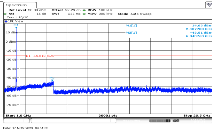
11B-CDD_Ant2_2437_1000~26500
