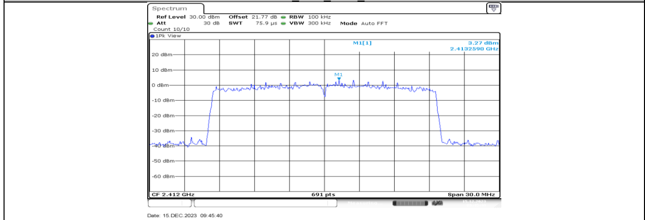
11AX20MIMO_Ant2_2412_0~Reference
