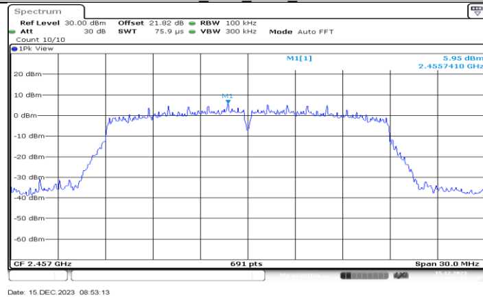
11N20MIMO_Ant2_2457_0~Reference
