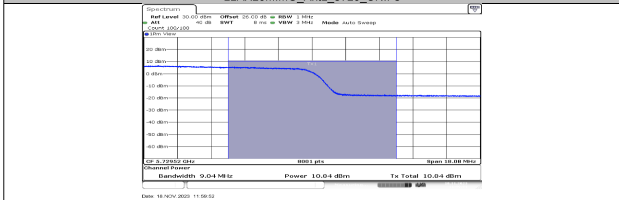
11AX20MIMO_Ant2_5720_UNII-3
