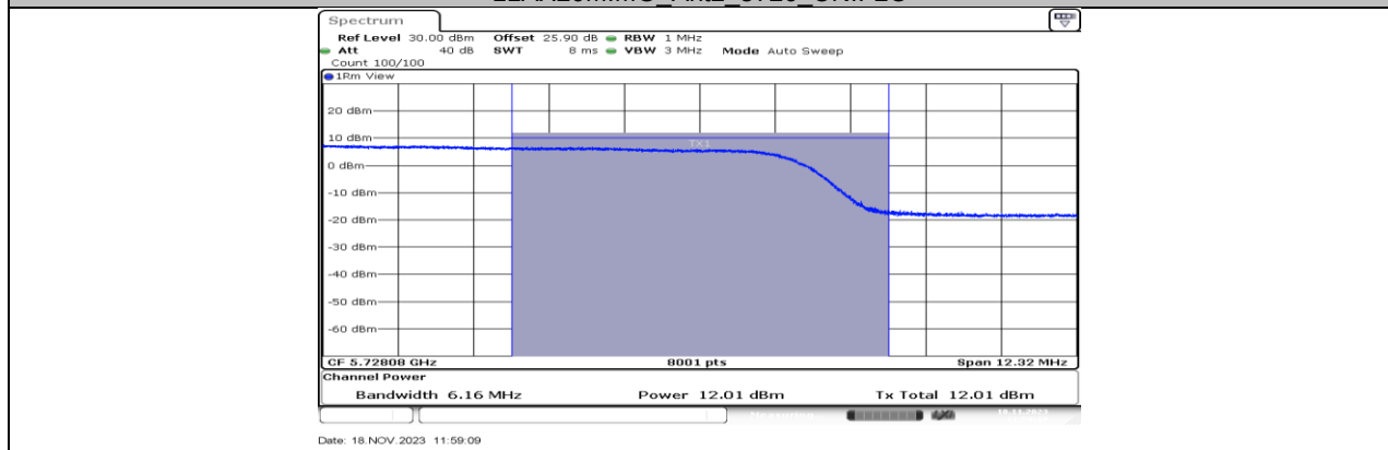
11AX20MIMO_Ant1_5720_UNII-3
