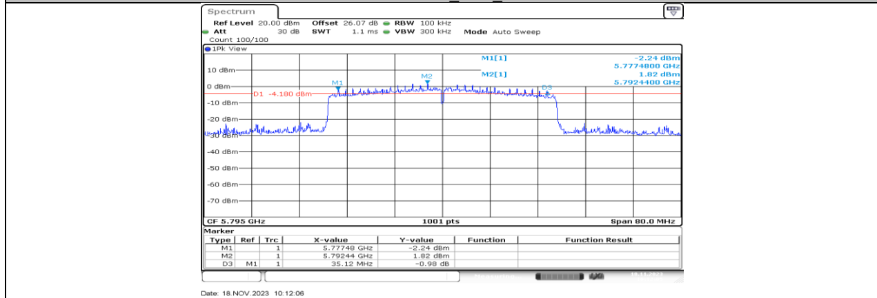
11AX40MIMO_Ant2_5795
