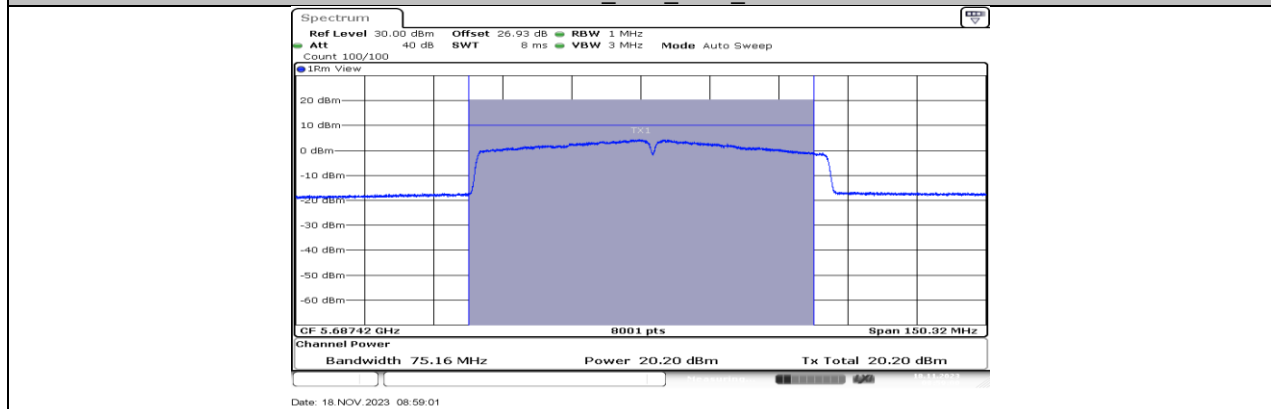
11AC80MIMO_Ant2_5690_UNII-2C
