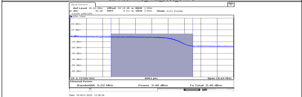
11AX80MIMO_Ant2_5690_UNII-3
