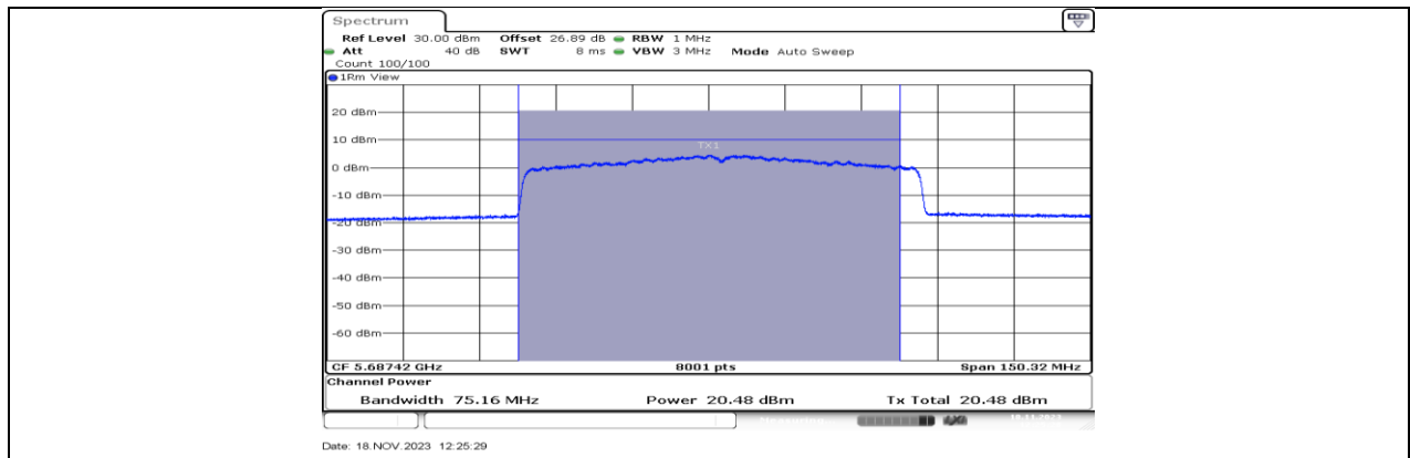
11AX80MIMO_Ant1_5690_UNII-2C
