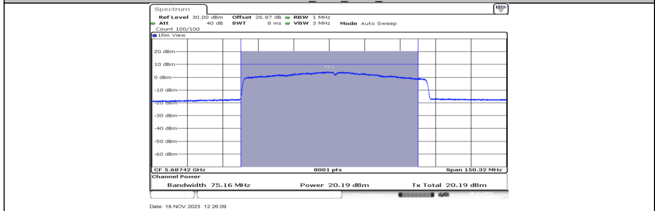
11AX80MIMO_Ant2_5690_UNII-2C
