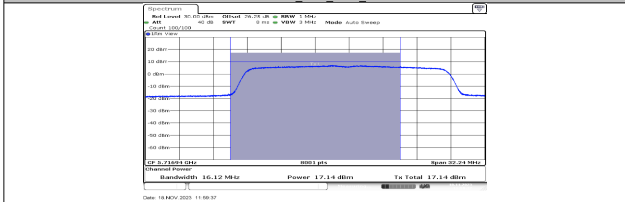
11AX20MIMO_Ant2_5720_UNII-2C
