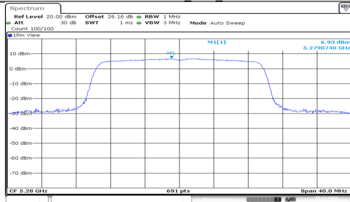
11AX20MIMO_Ant1_5280
