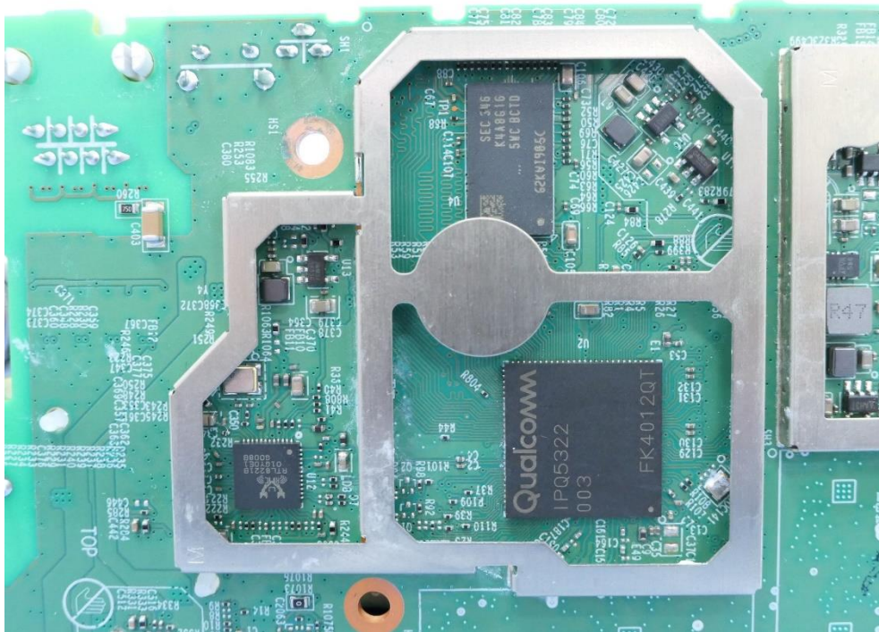
(8) EUT Photo
