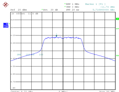
CH144
