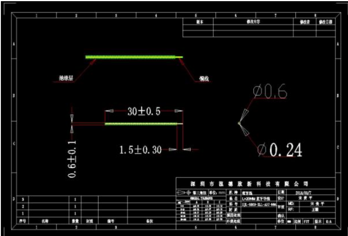
蓝牙线 31.5mm
