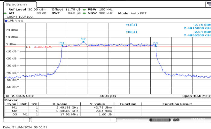
SRD 20MHz_Ant1_2410.5
