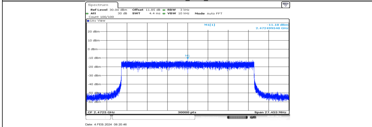
SRD 20MHZ_Ant2_2472.5
