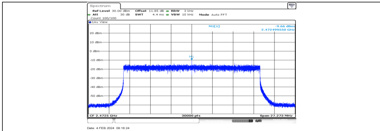
SRD 20MHZ_Ant1_2472.5
