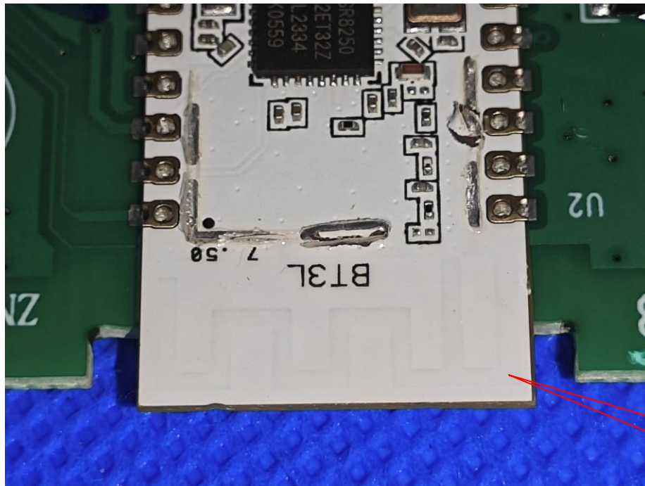
BLE antenna
