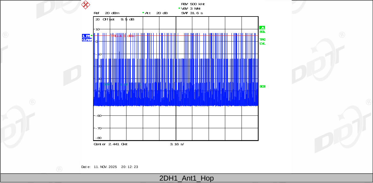
2DH1_Ant1_Hop
