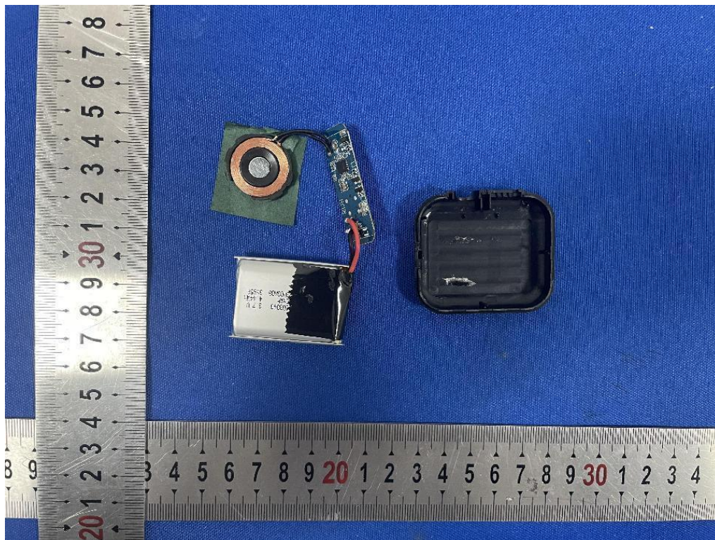
Internal-2
