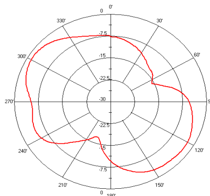
AN3216 E-Plane
