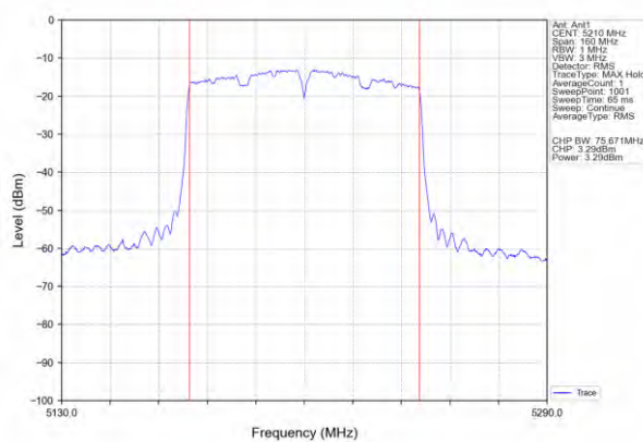
5210MHz
