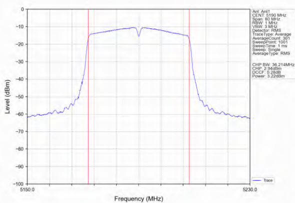
5190MHz
