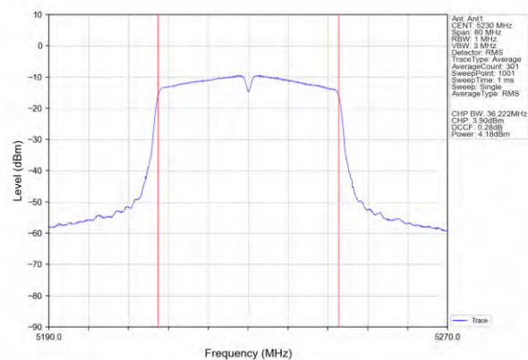
5230MHz
