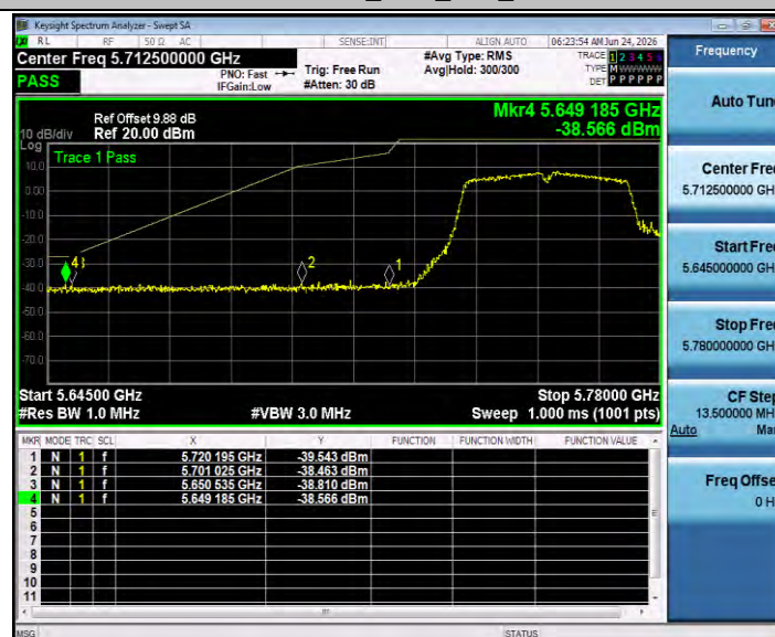
11N40ISO_Ant3_Low_5755
