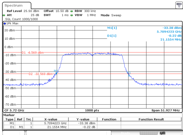
802.11ac20_5720MHz_Chain 0
