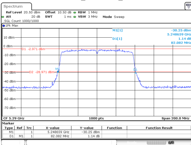
802.11ac80_5290MHz_Chain 1
