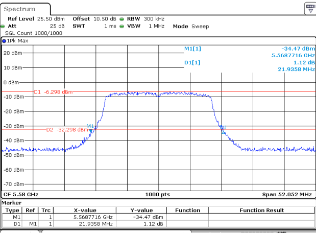
802.11ac20_5580MHz_Chain 1
