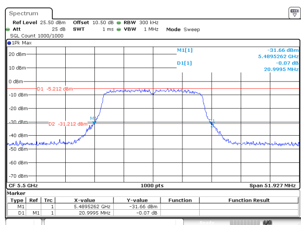
802.11ac20_5500MHz_Chain 1
