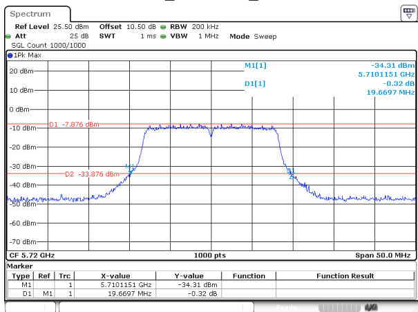
802.11a_5720MHz_Chain 1
