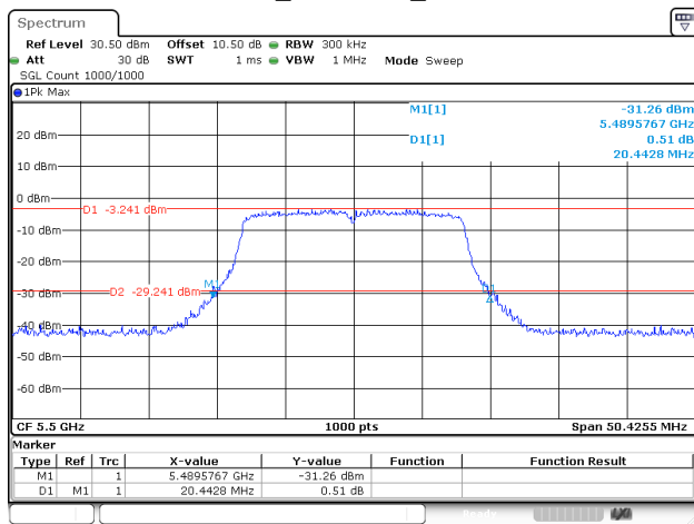
802.11a_5500MHz_Chain 1
