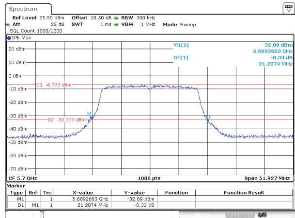
802.11ac20_5700MHz_Chain 0
