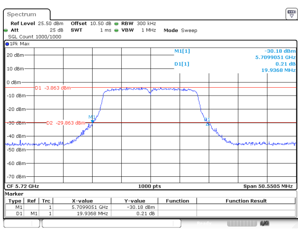
802.11a_5720MHz_Chain 0
