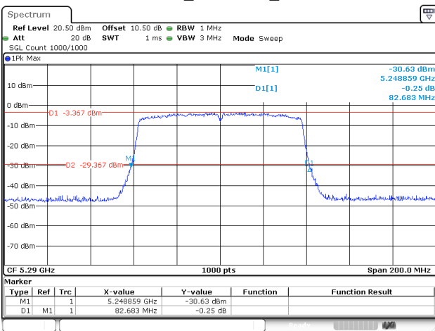
802.11ac80_5290MHz_Chain 0
