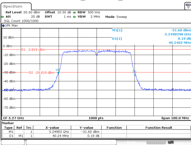
802.11ac40_5270MHz_Chain 1
