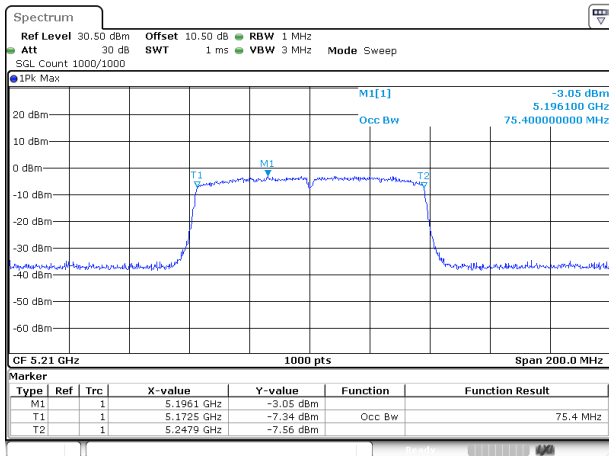
802.11ac80_5210MHz_Chain 0
