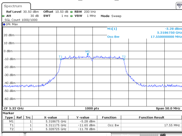
802.11ac20_5320MHz_Chain 0
