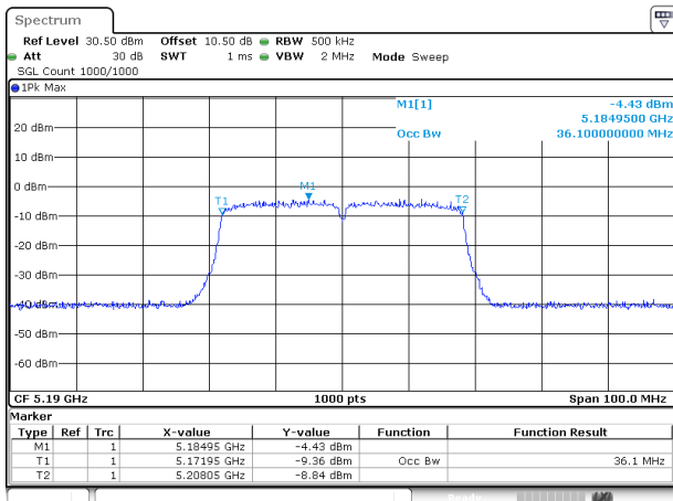
802.11ac40_5190MHz_Chain 1
