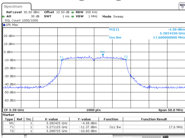
802.11ac20_5280MHz_Chain 1
