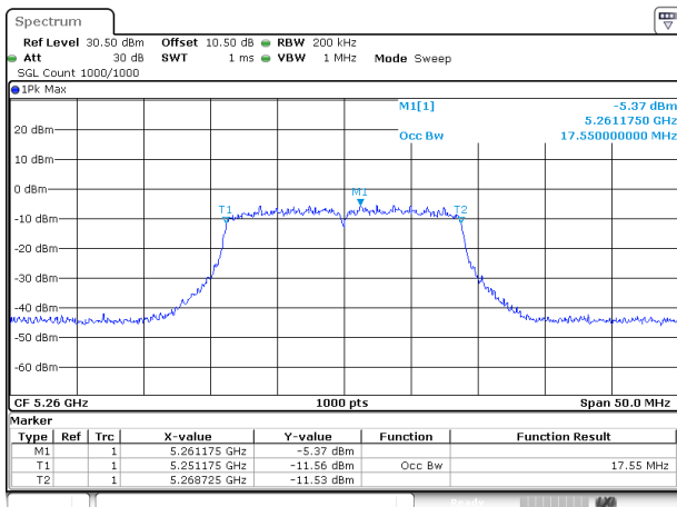
802.11ac20_5260MHz_Chain 0
