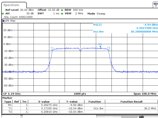
802.11ac40_5190MHz_Chain 0
