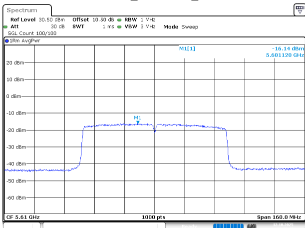
802.11ac80_5610MHz_Chain 1
