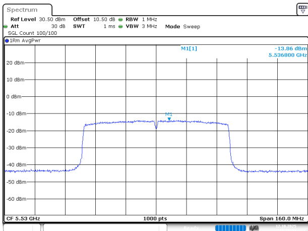
802.11ac80_5530MHz_Chain 0
