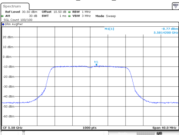
802.11ac20_5580MHz_Chain 1
