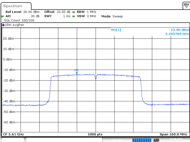
802.11ac80_5610MHz_Chain 0
