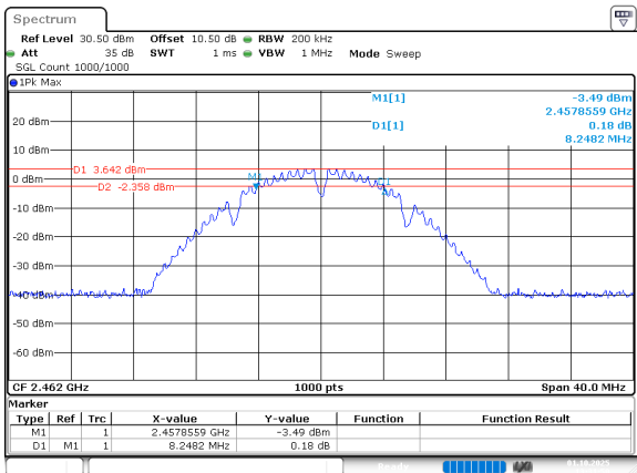
802.11b_2462MHz_Chain 1
