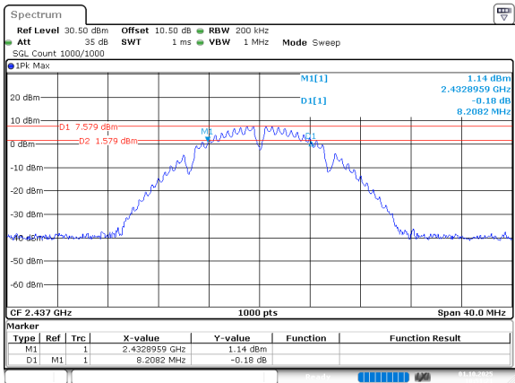
802.11b_2437MHz_Chain 0
