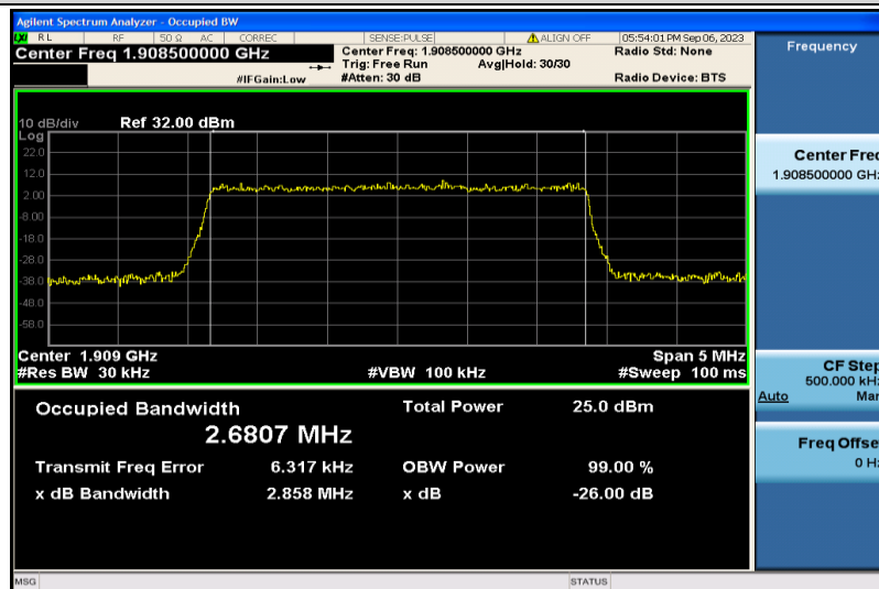
Band2-3MHz-QPSK-19185-15RB#0-2.6807
