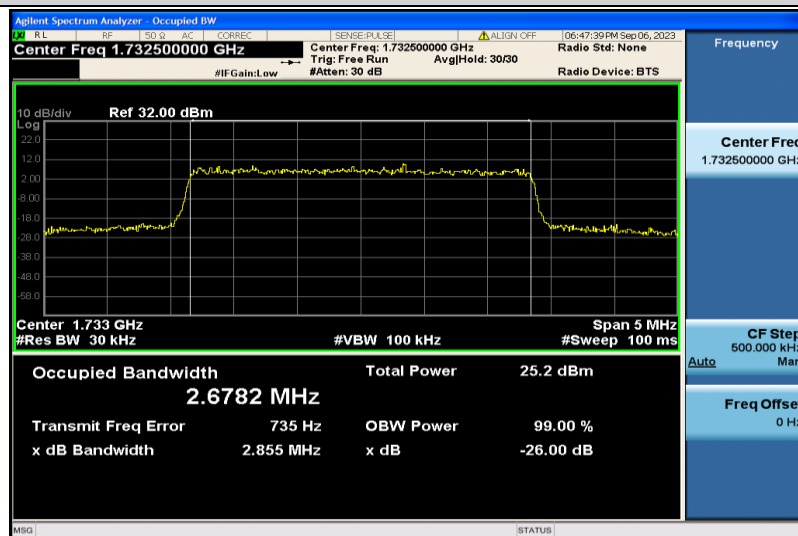
Band4-3MHz-QPSK-17325-15RB#0-2.6782
