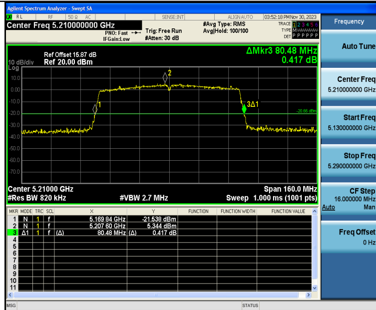
11AC80SISO-Ant1-5210
