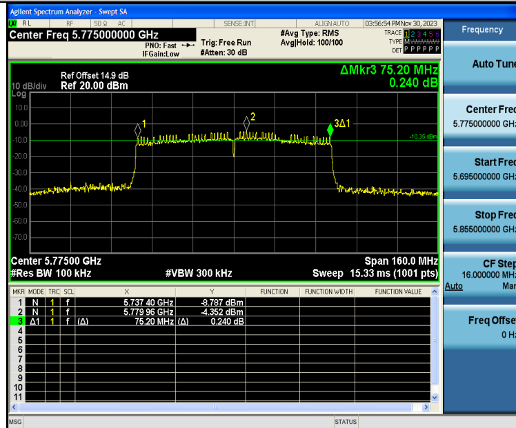
11AC80SISO-Ant1-5775-PASS
