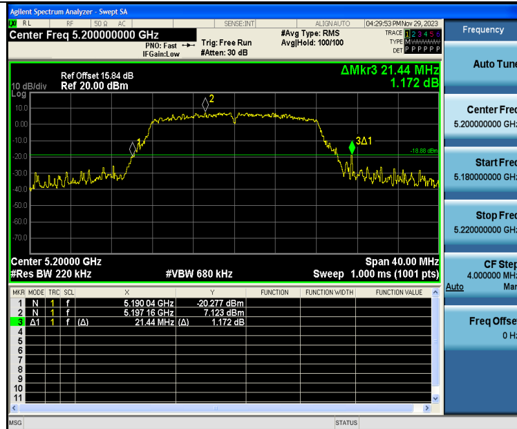
11A-Ant1-5200
